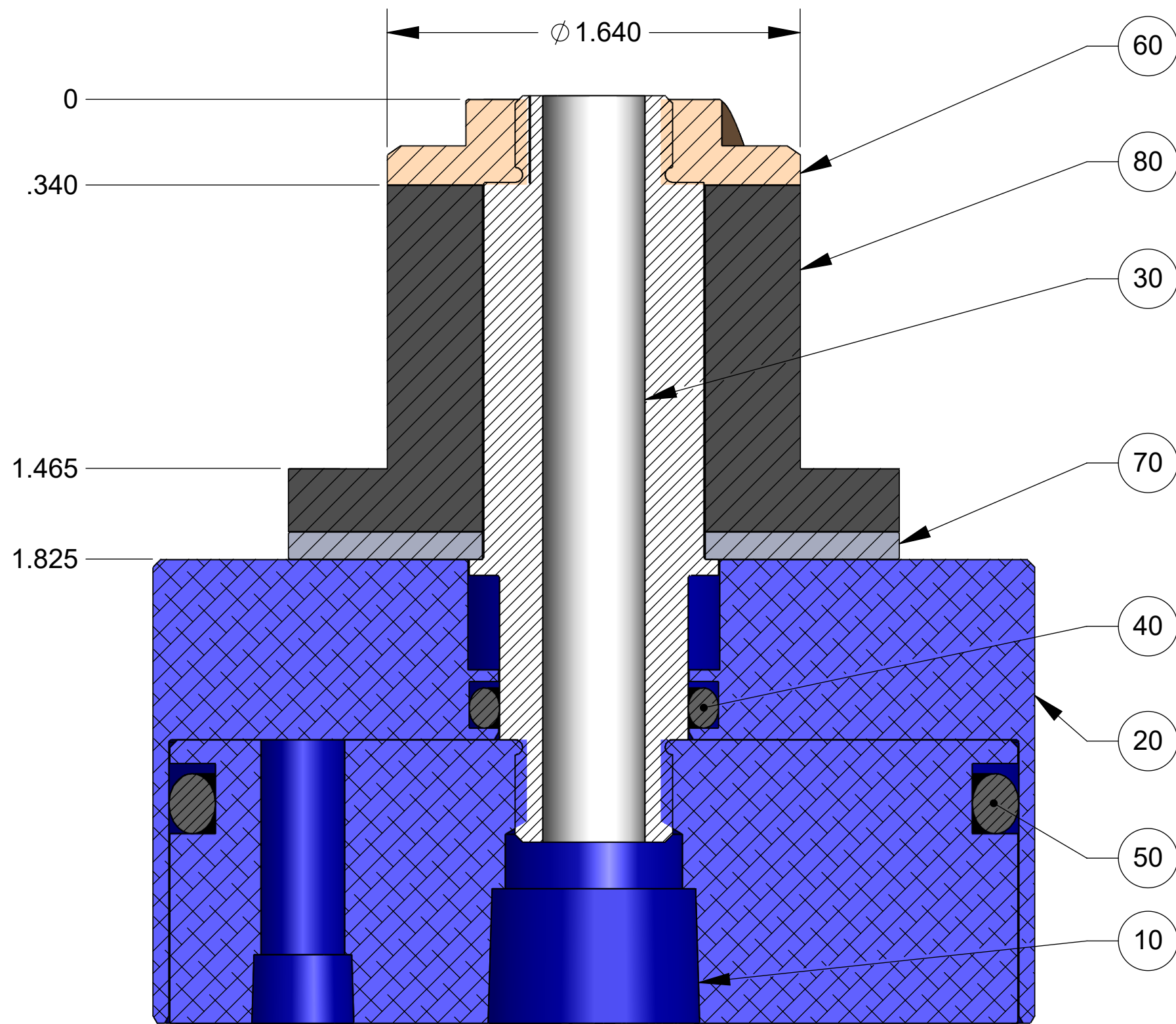
SECTION A-A SCALE 2 : 1
