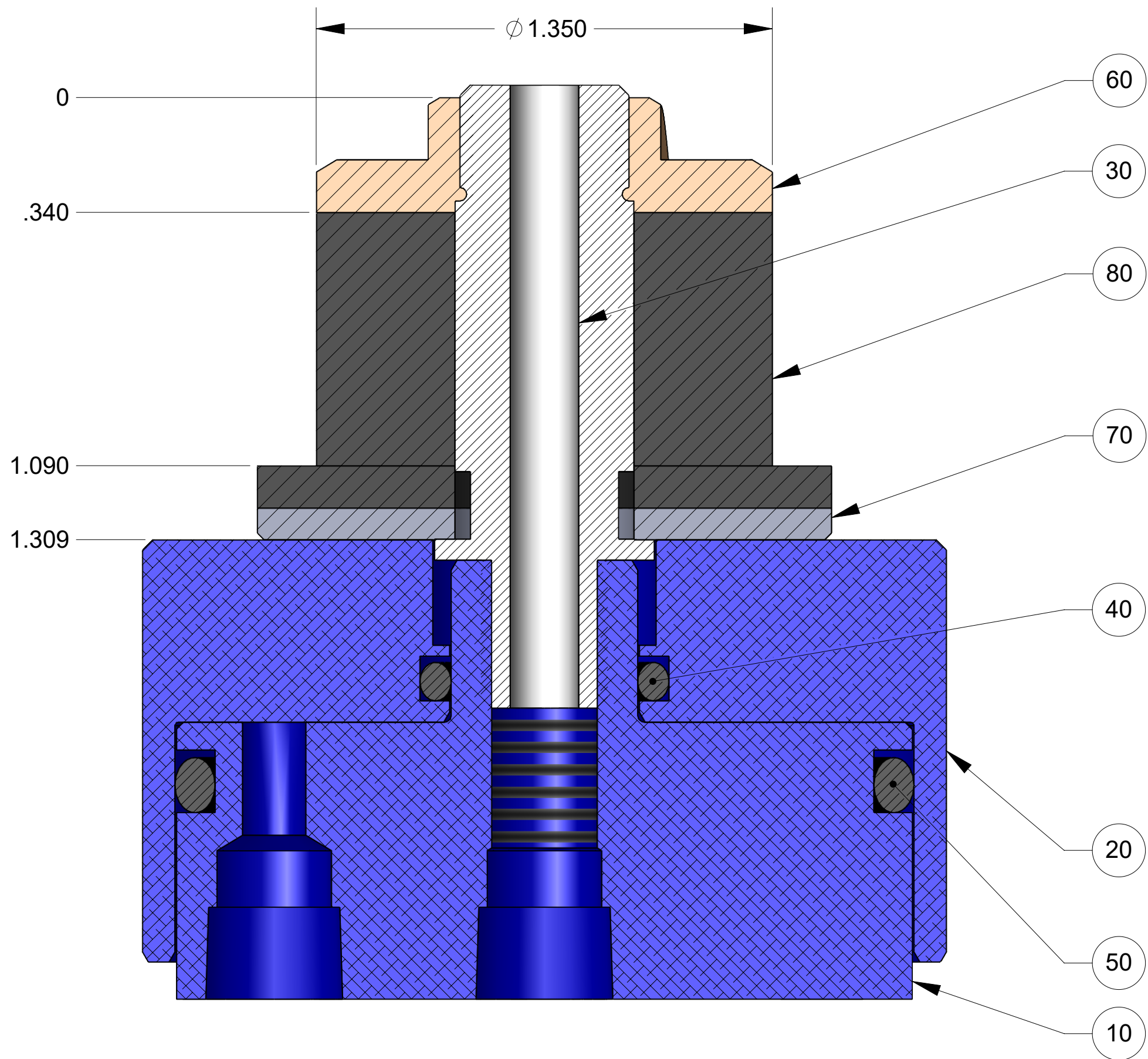
SECTION A-A SCALE 3 : 1
