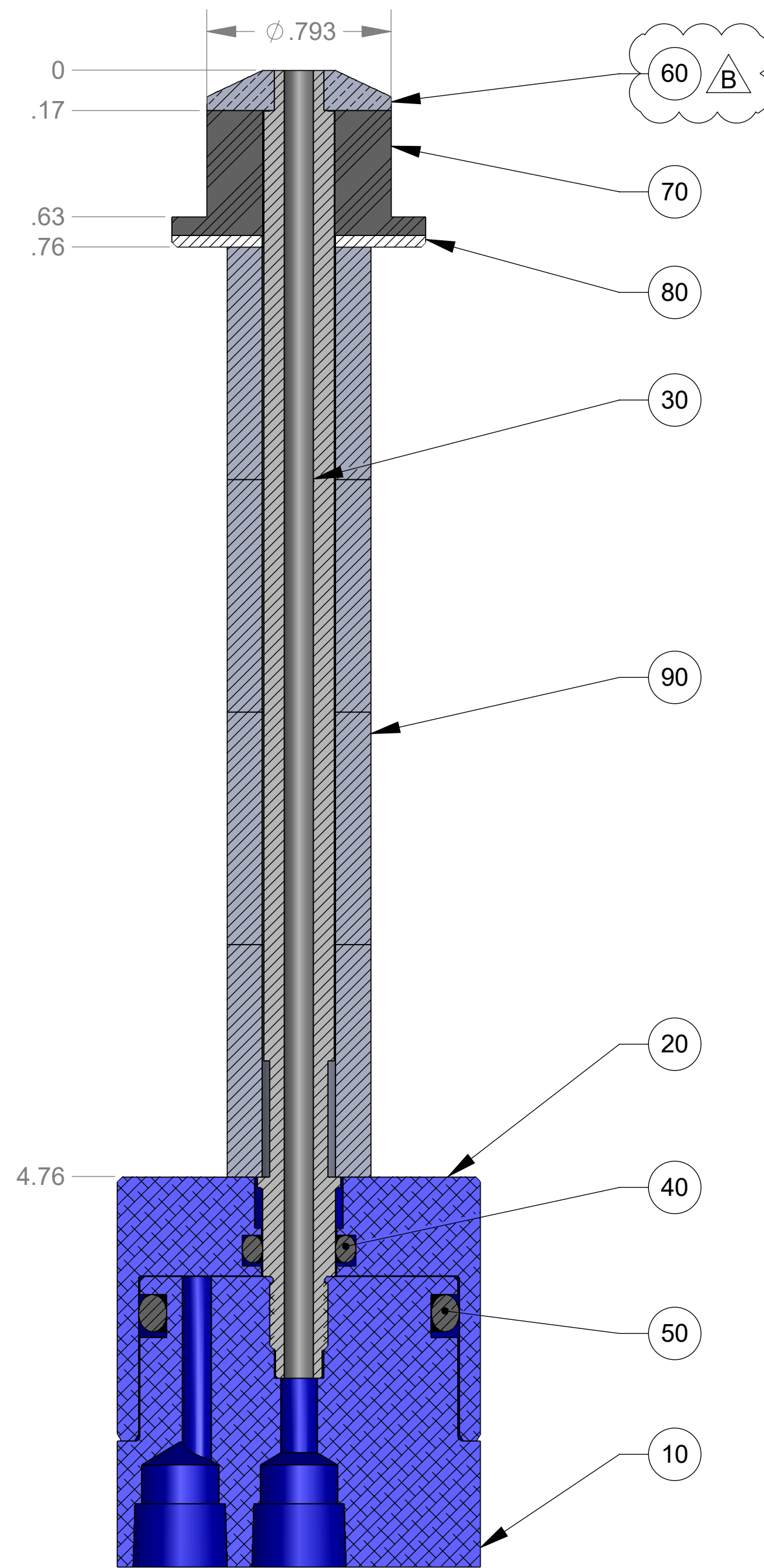
SECTION A-A
