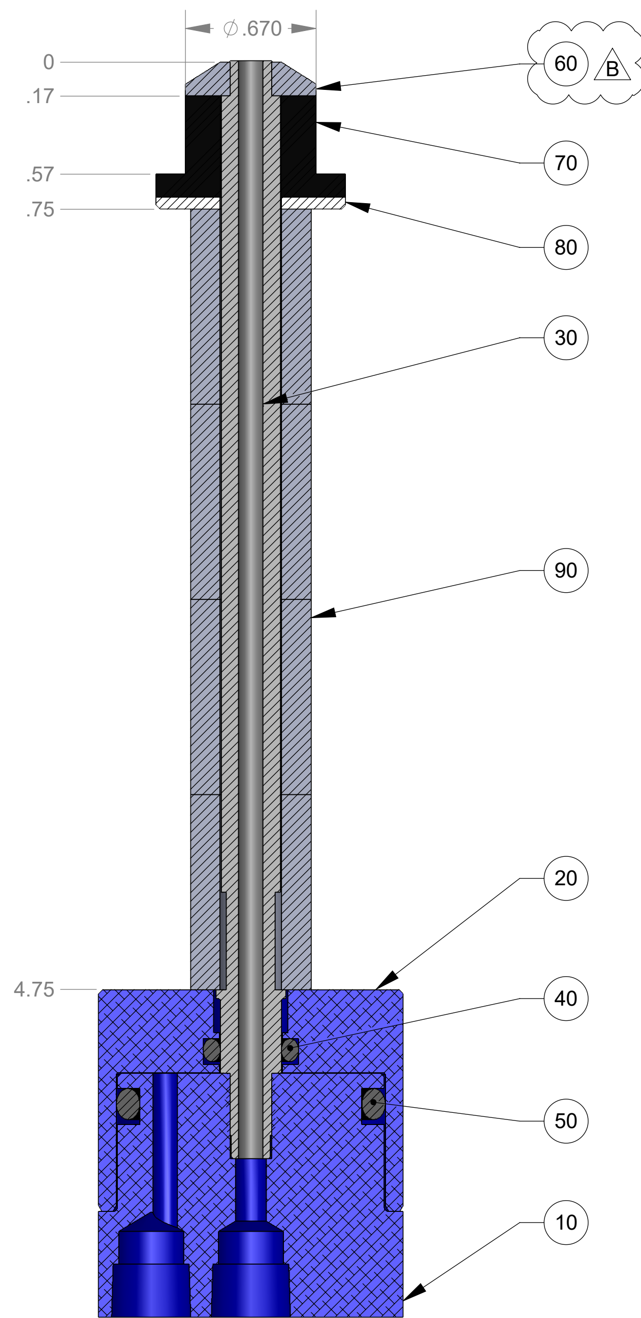
SECTION A-A
