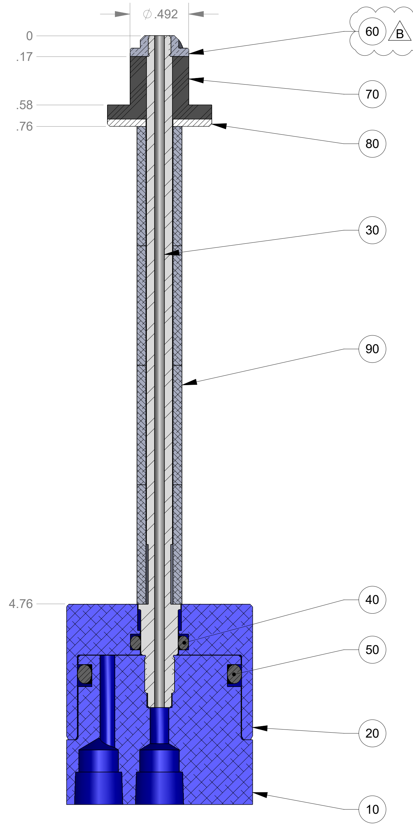
SECTION A-A
