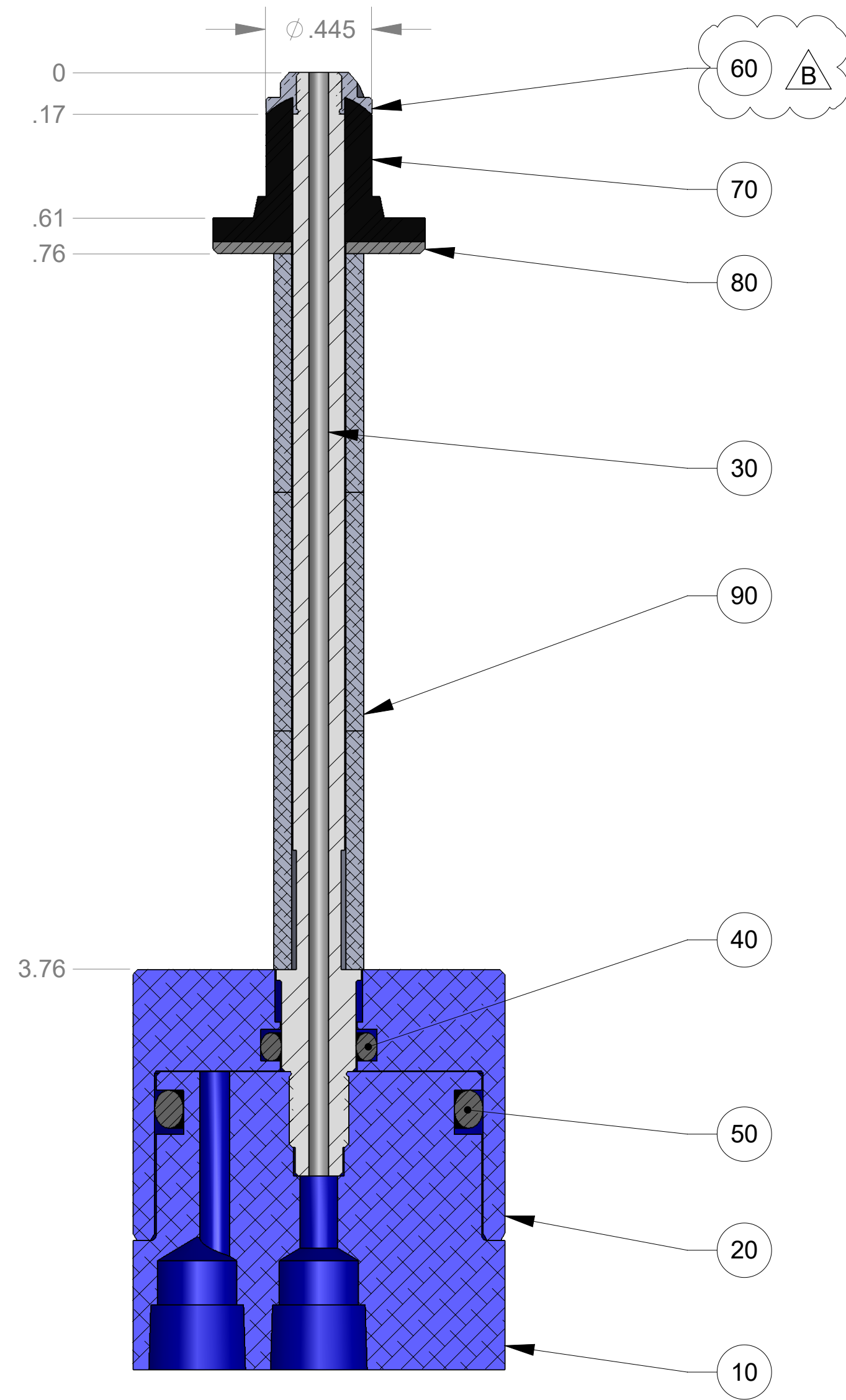
SECTION A-A
