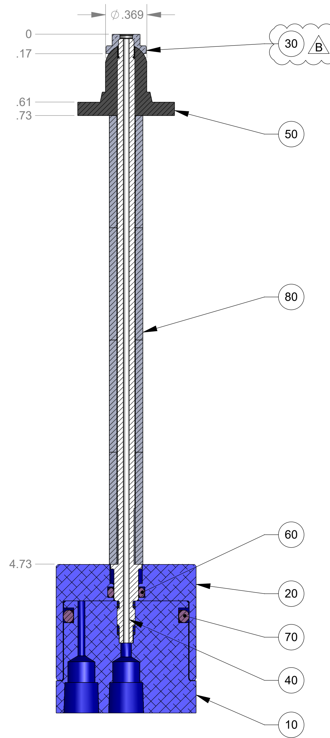
SECTION A-A
