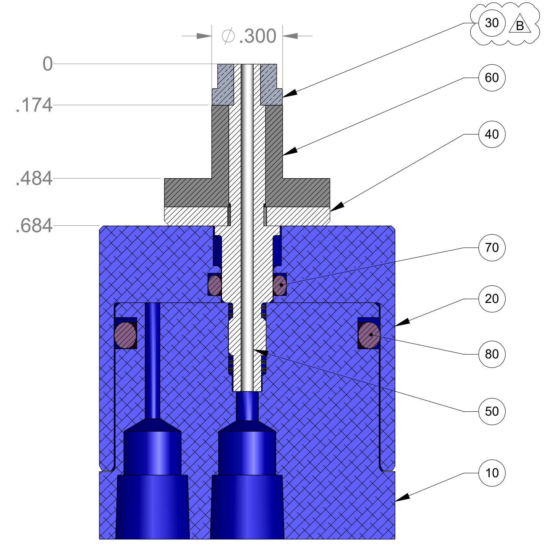
SECTION A-A SCALE 4 : 1
