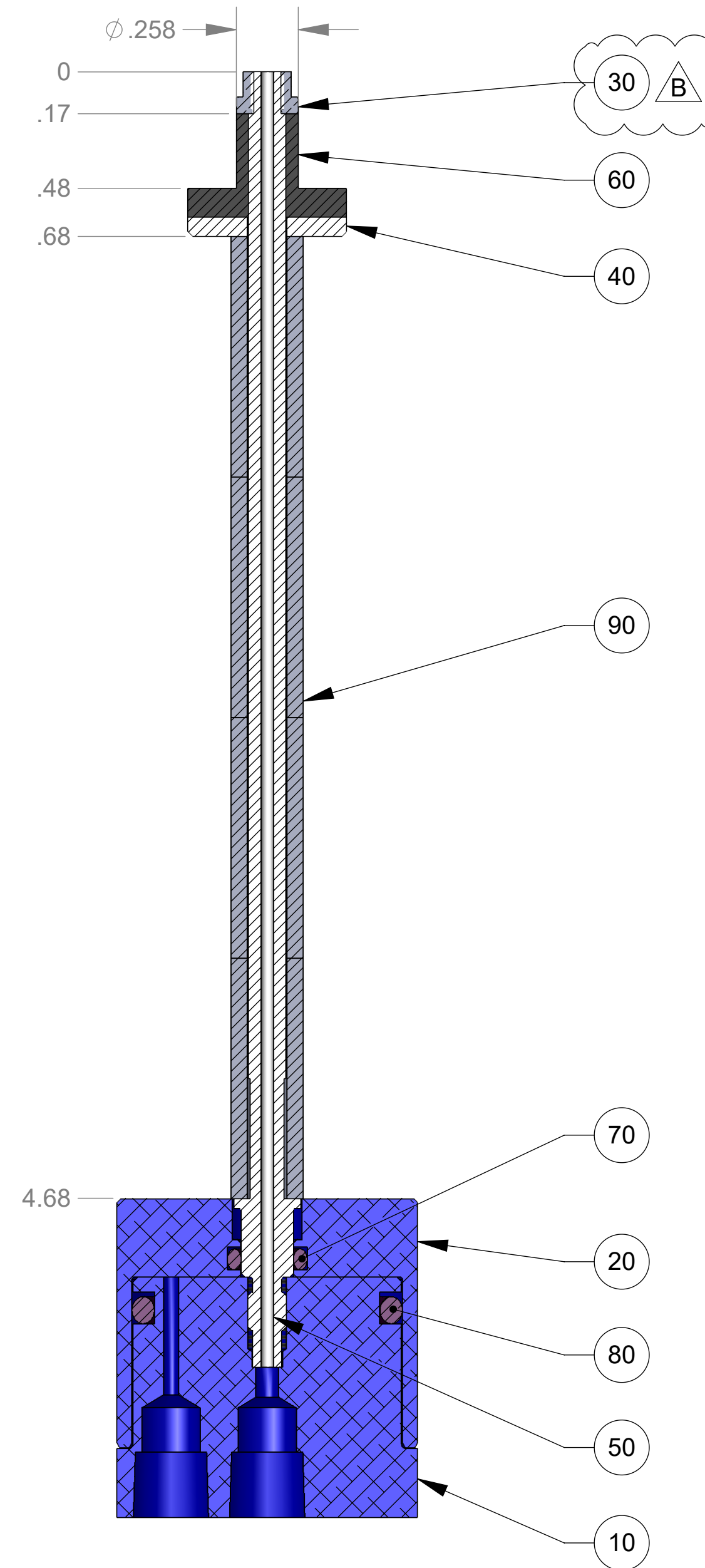
SECTION A-A
