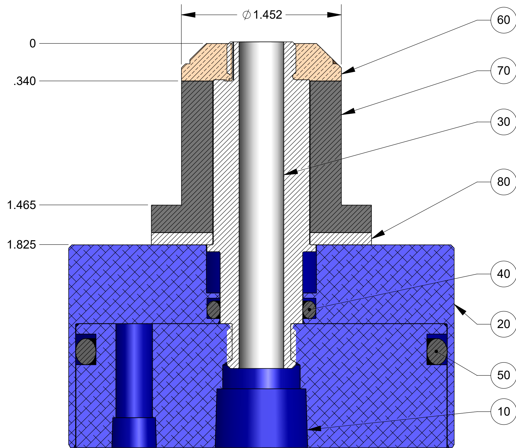
SECTION A-A SCALE 2 : 1
