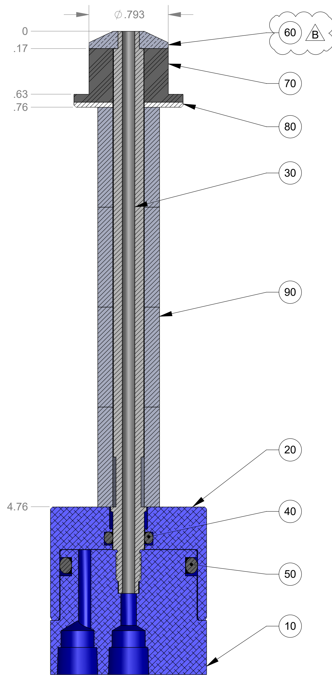
SECTION A-A
