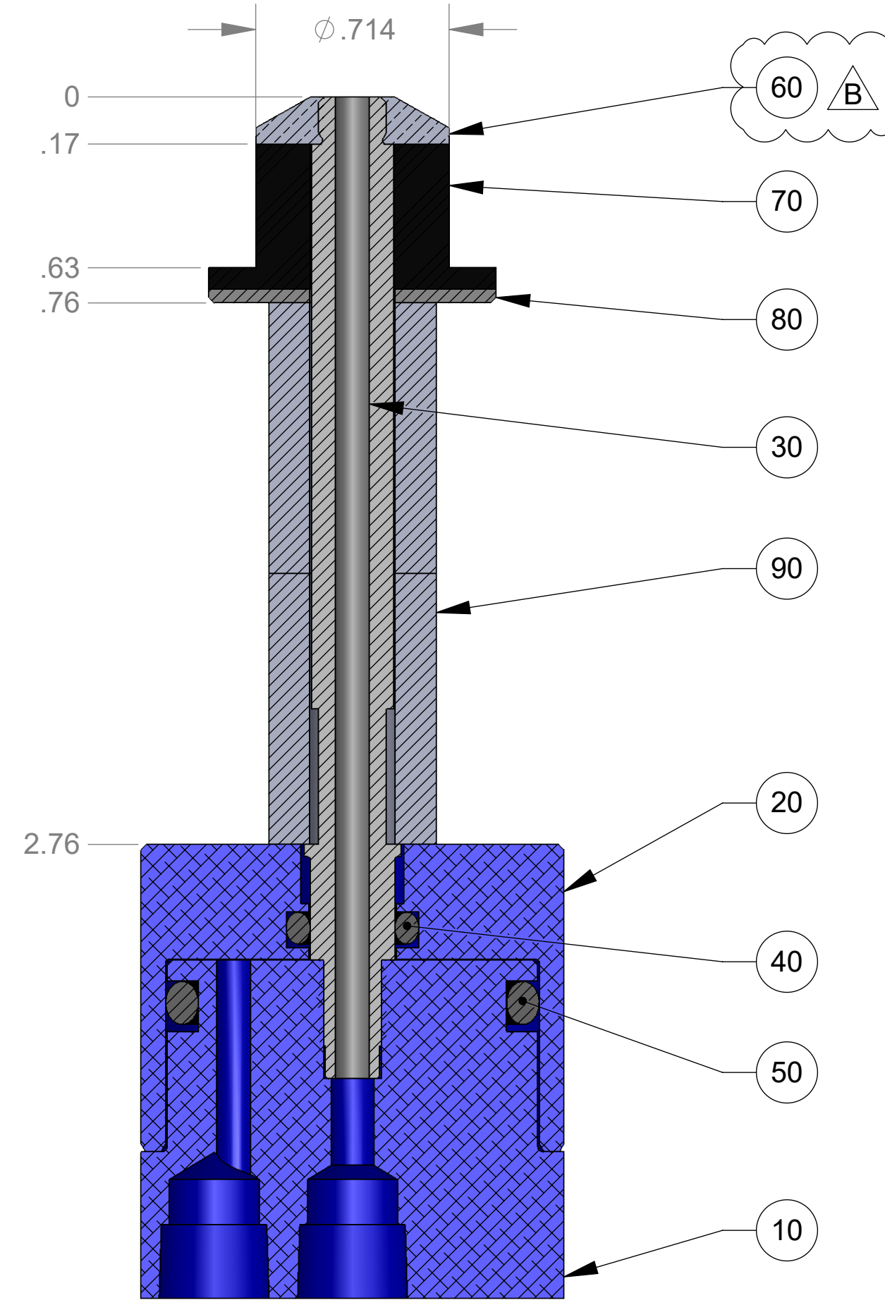
SECTION A-A
