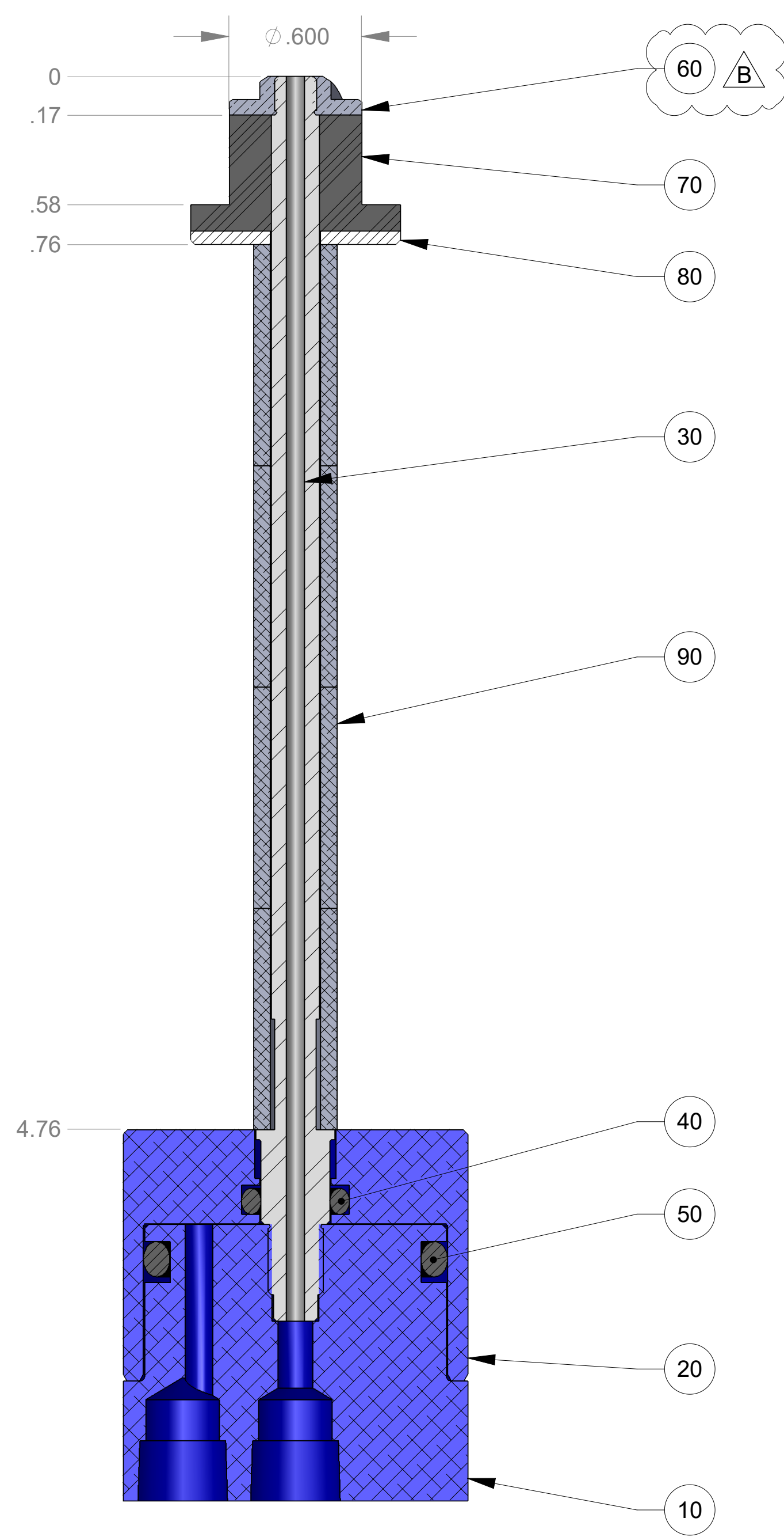
SECTION A-A
