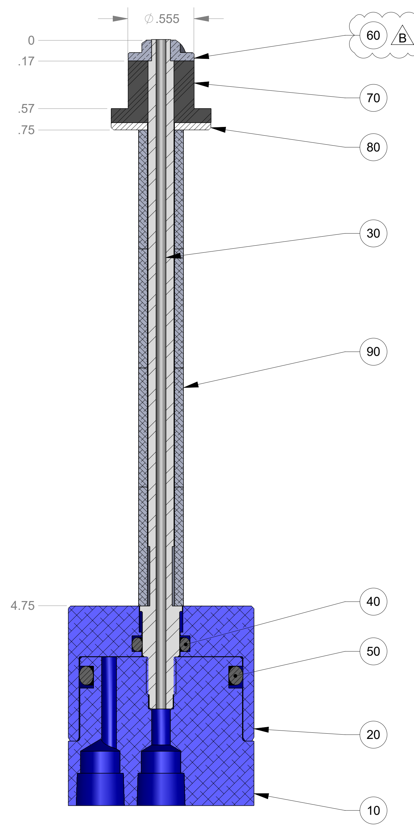
SECTION A-A
