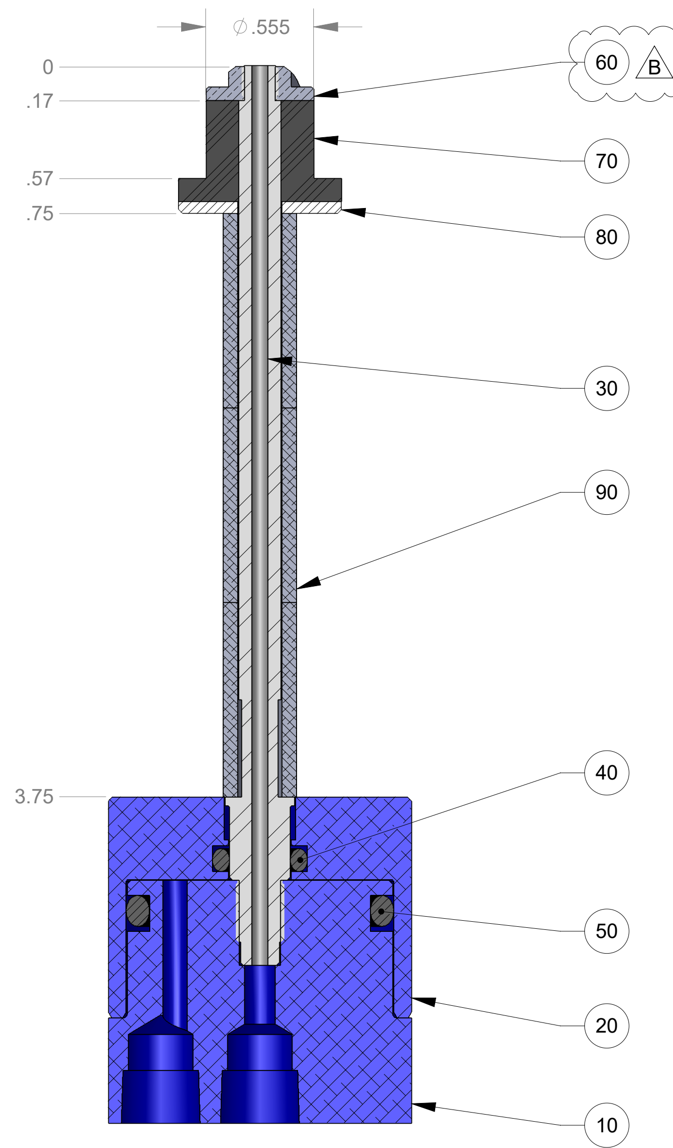
SECTION A-A
