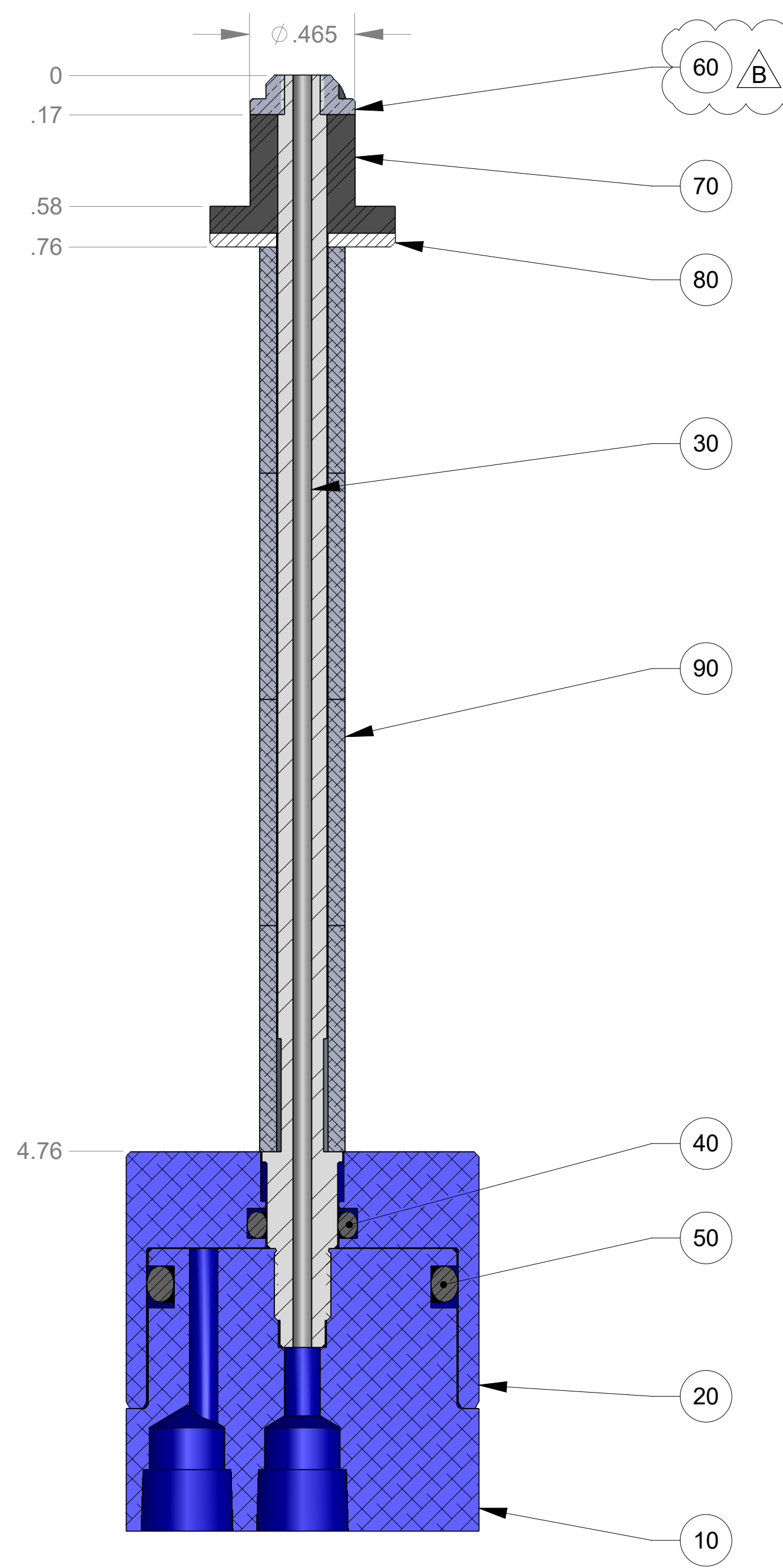
SECTION A-A
