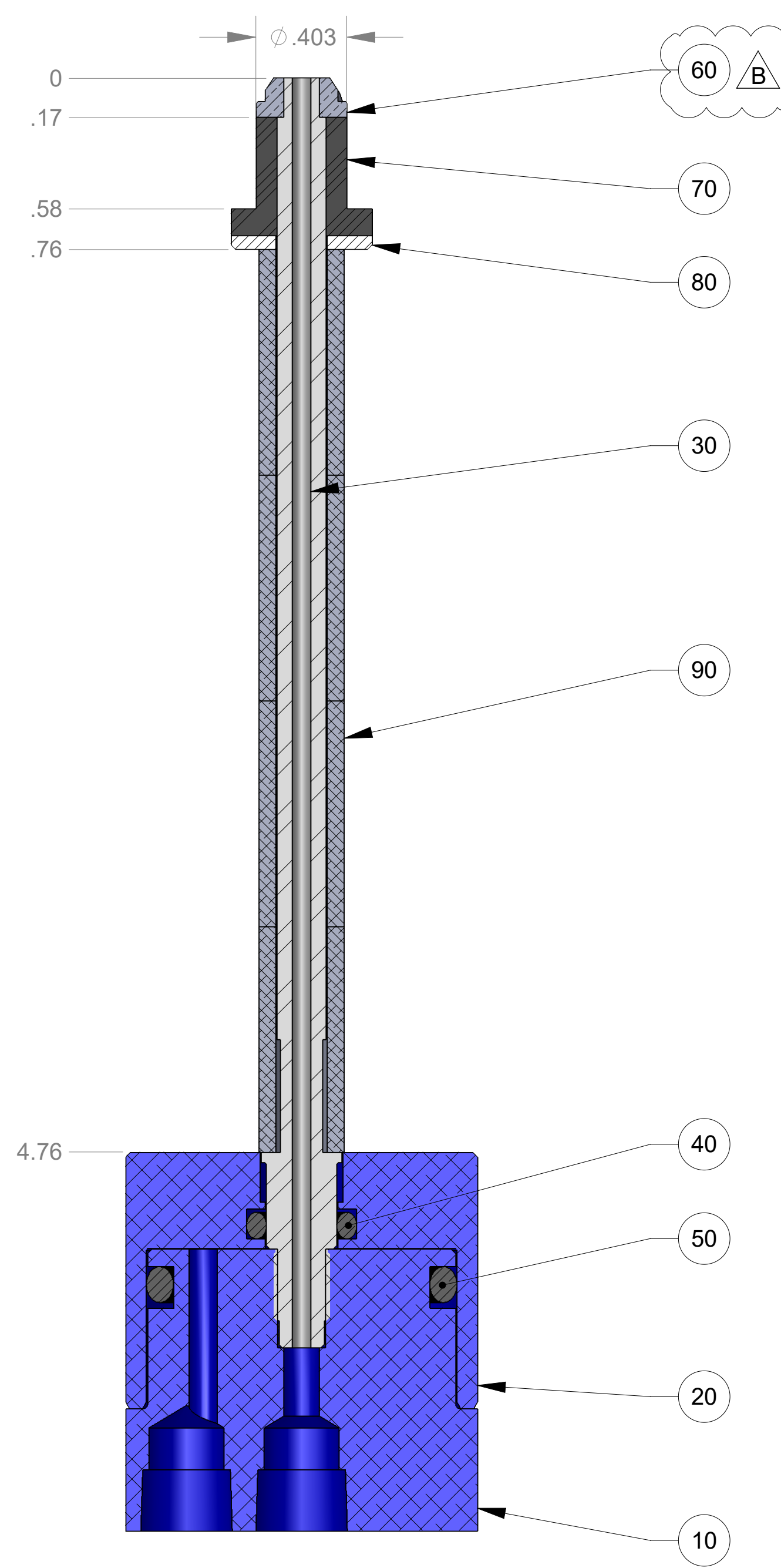
SECTION A-A
