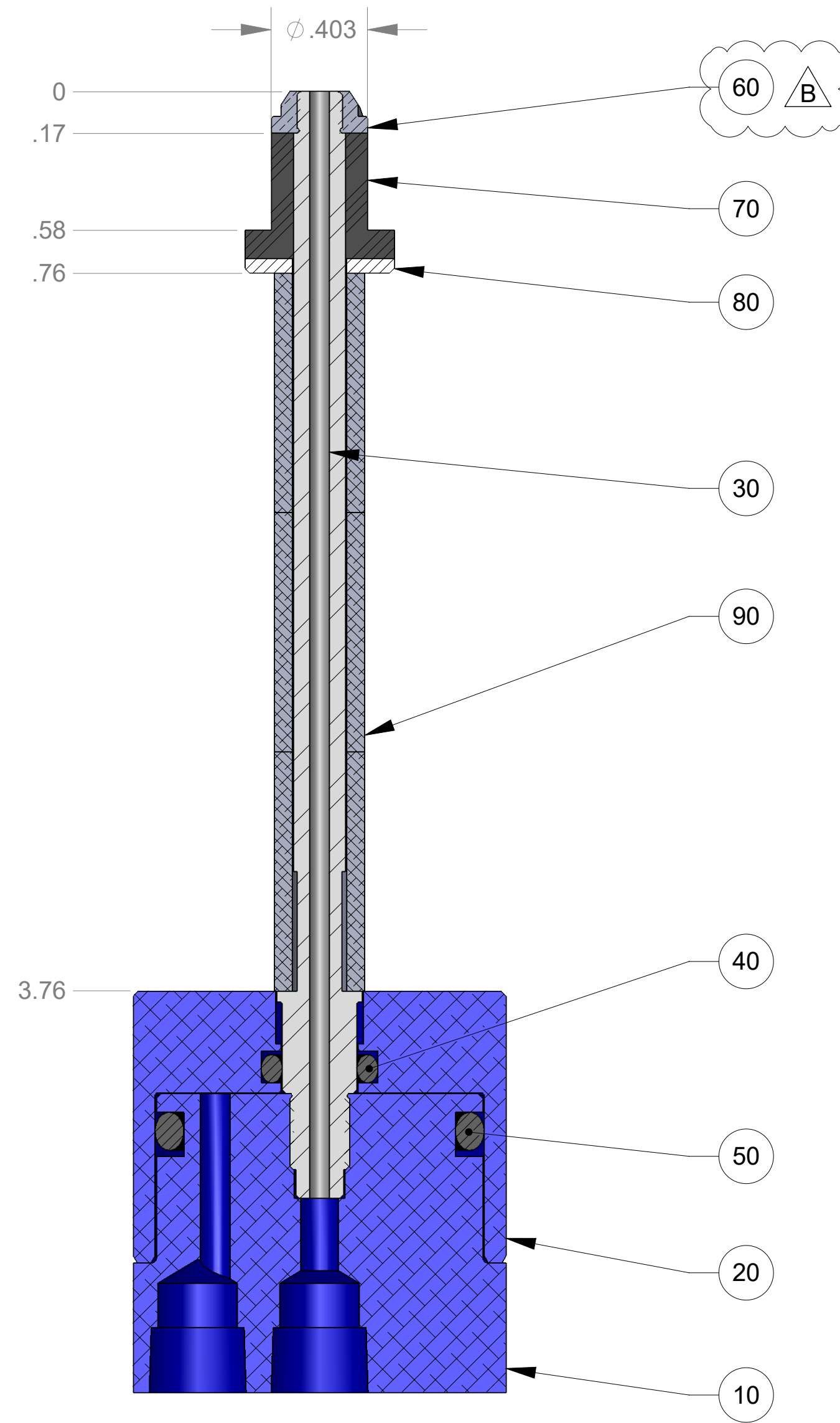
SECTION A-A
