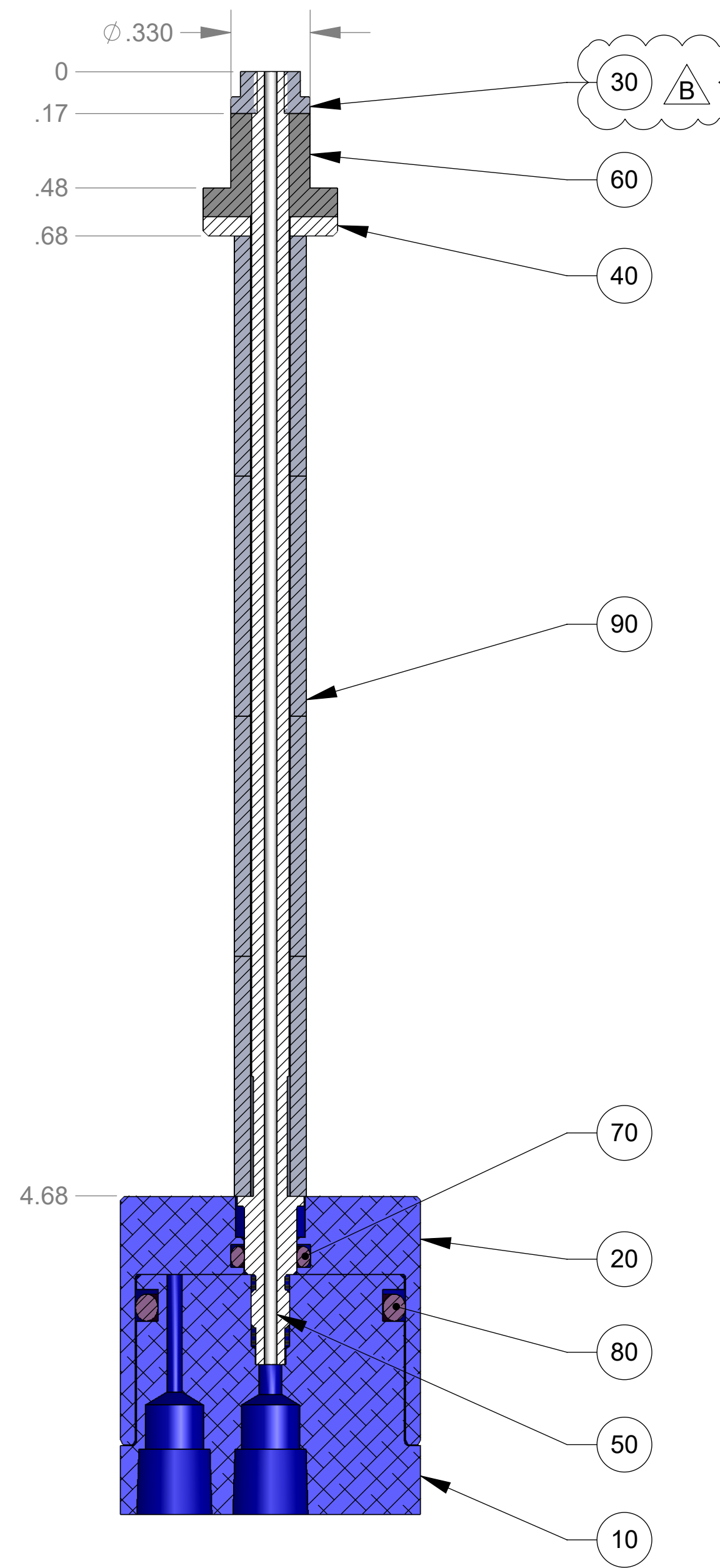
SECTION A-A
