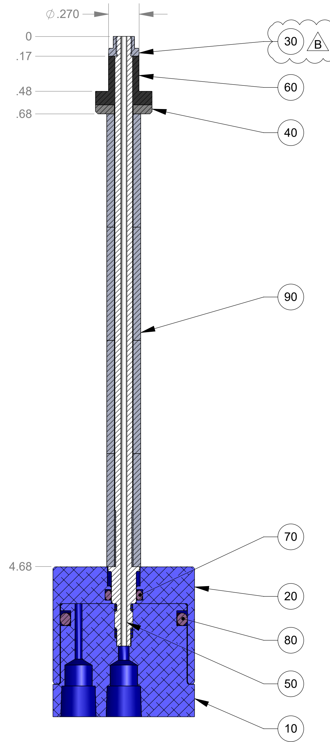
SECTION A-A
