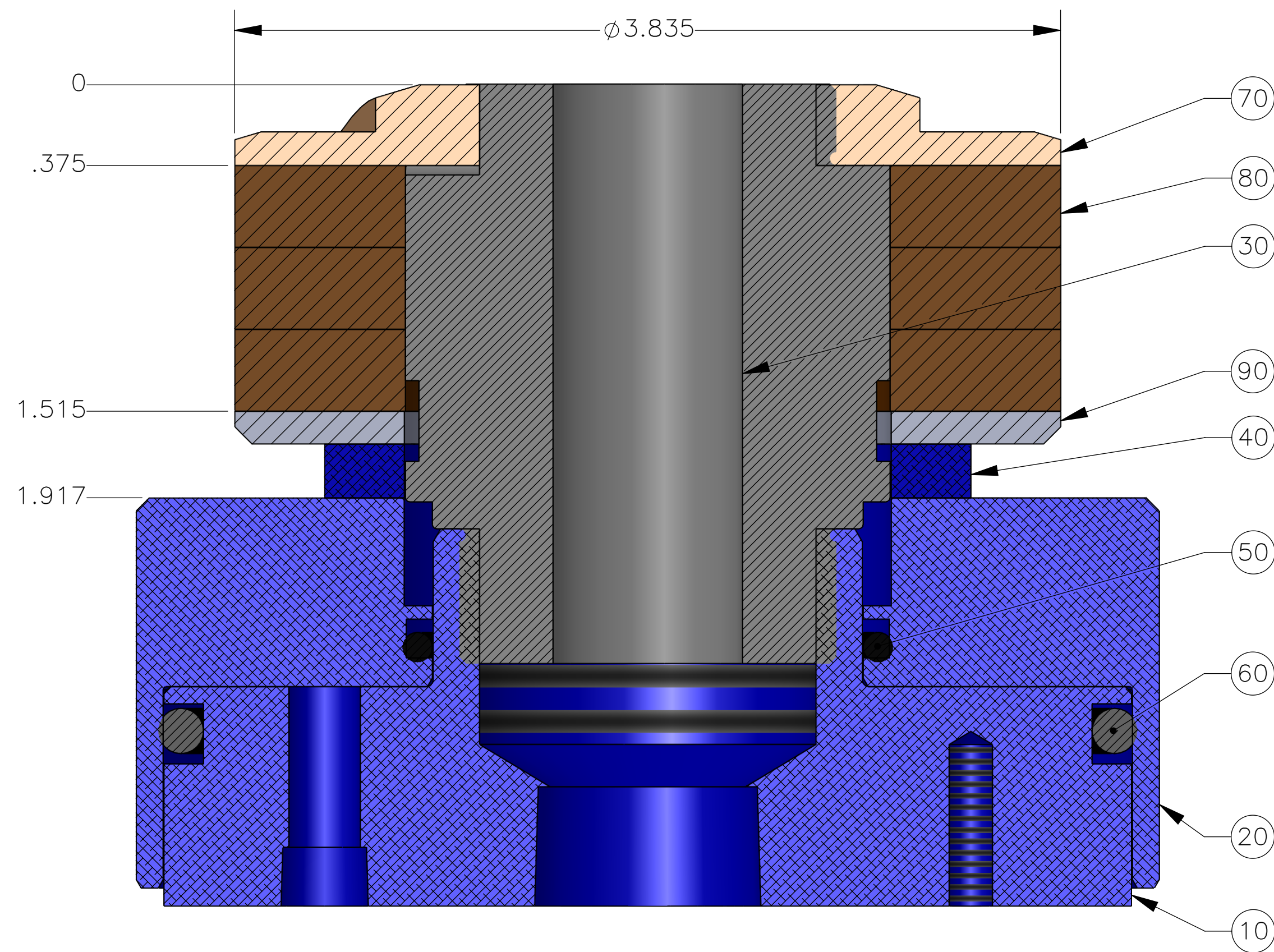
SECTION A-A SCALE 2 : 1
