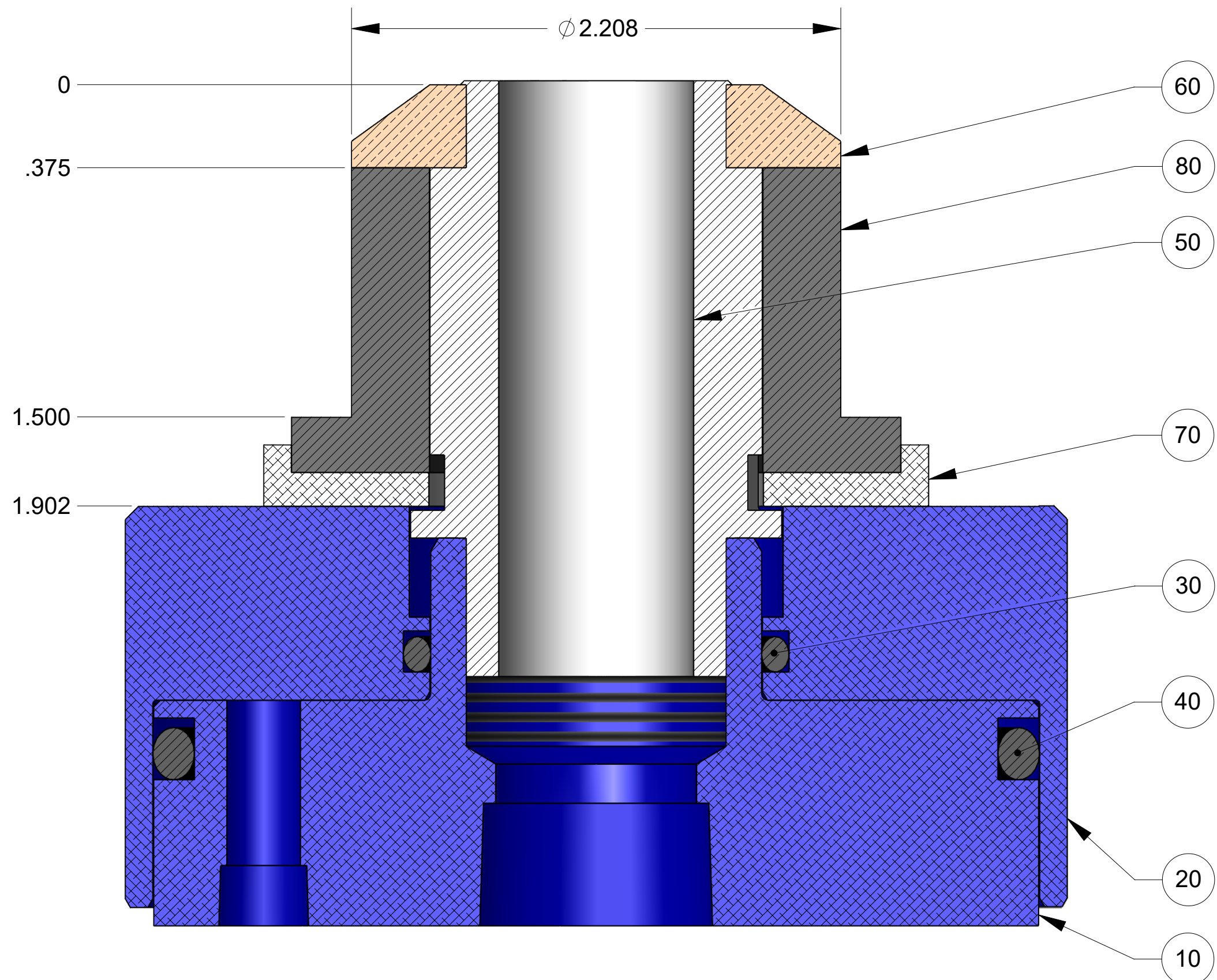
SECTION A-A SCALE 2 : 1
