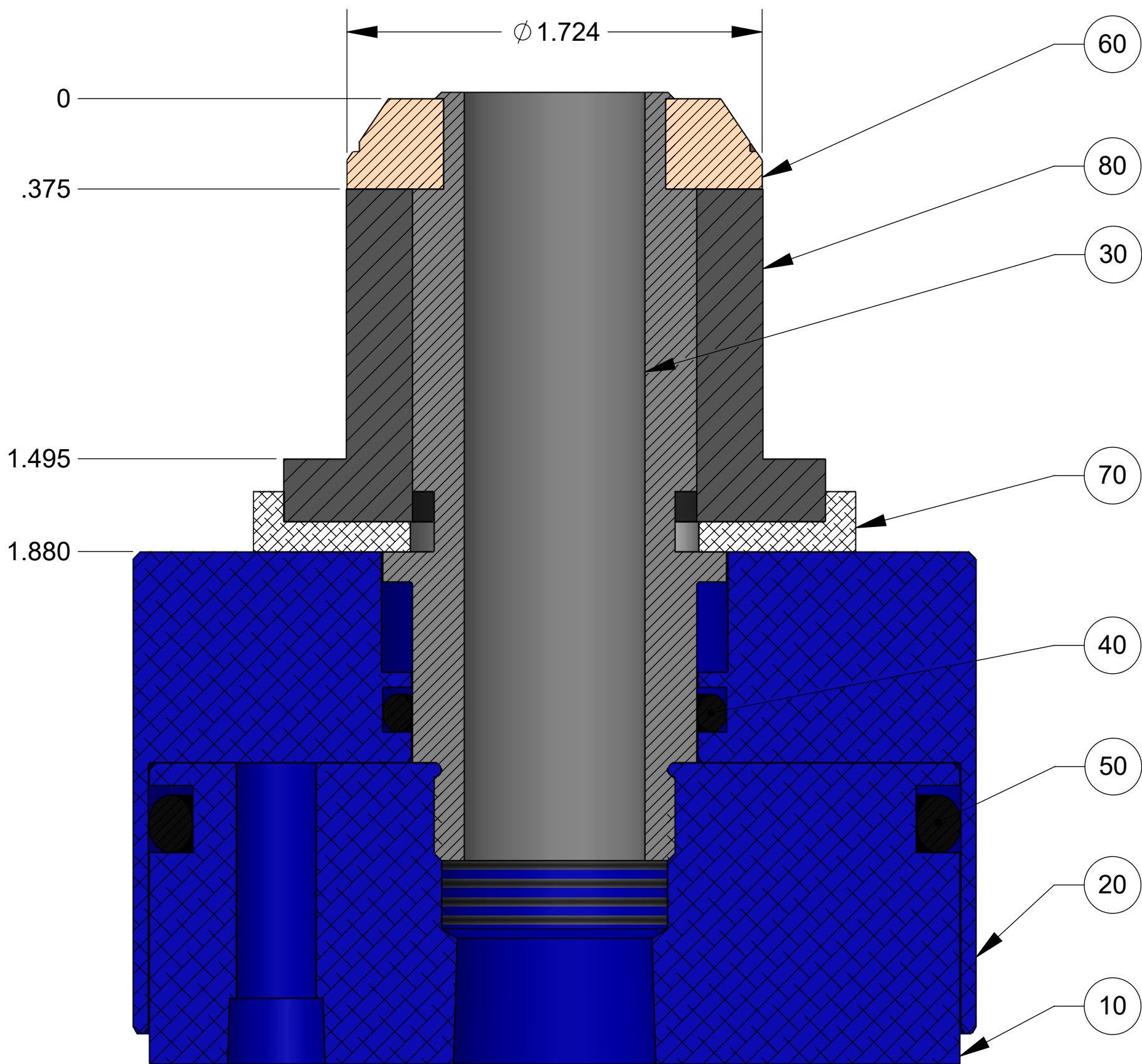
SECTION A-A SCALE 2 : 1
