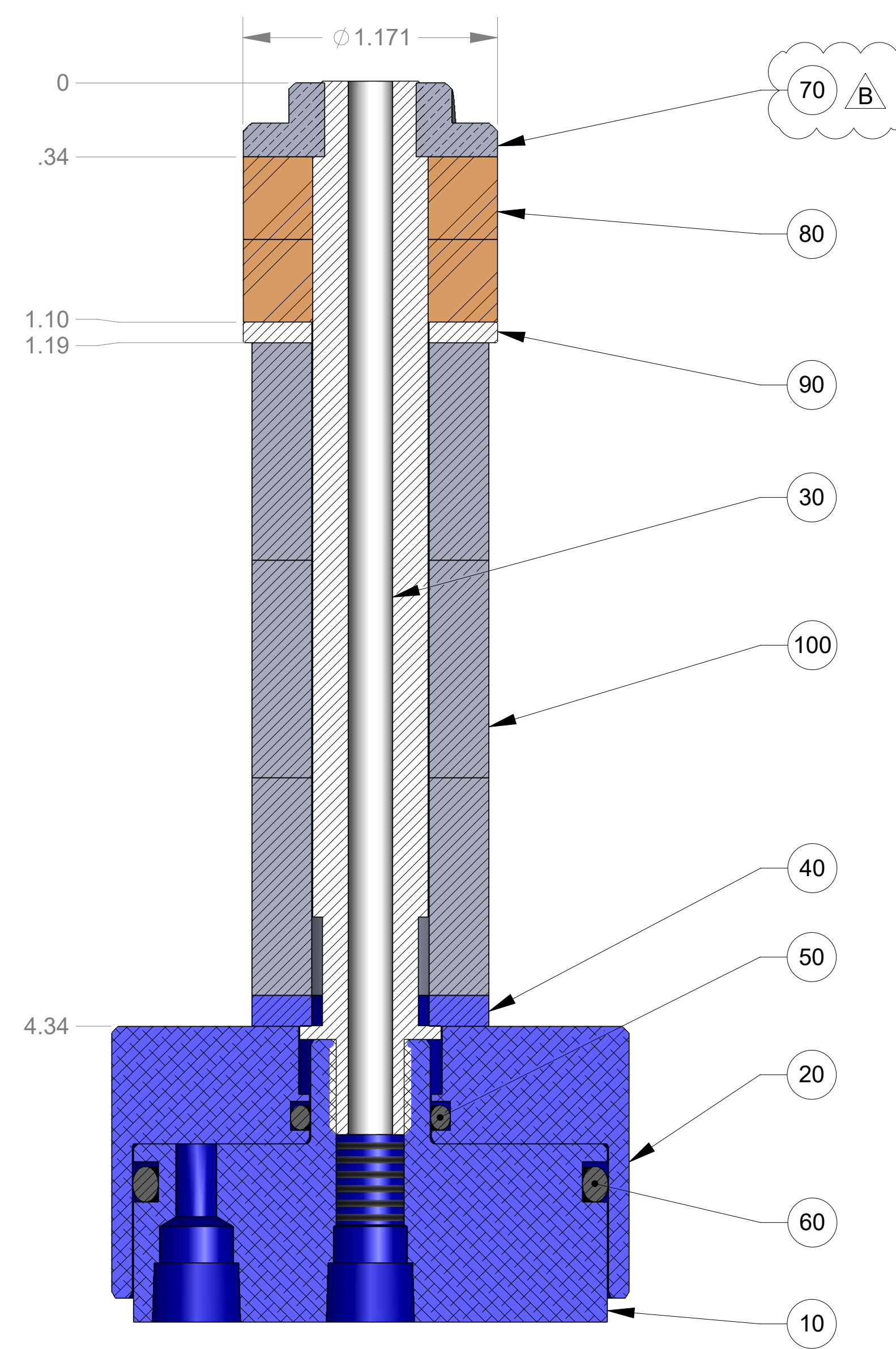
SECTION A-A
