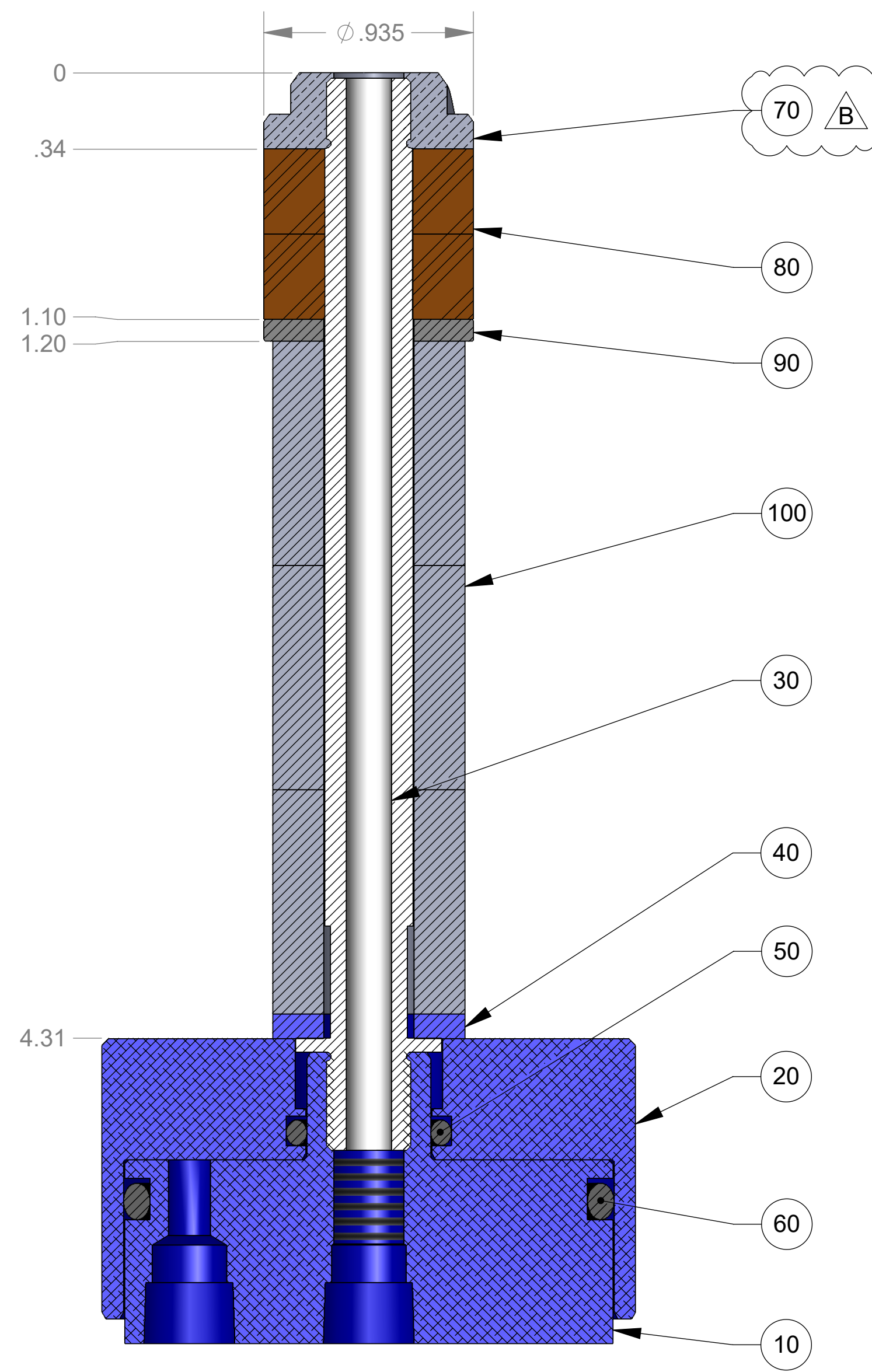
SECTION A-A
