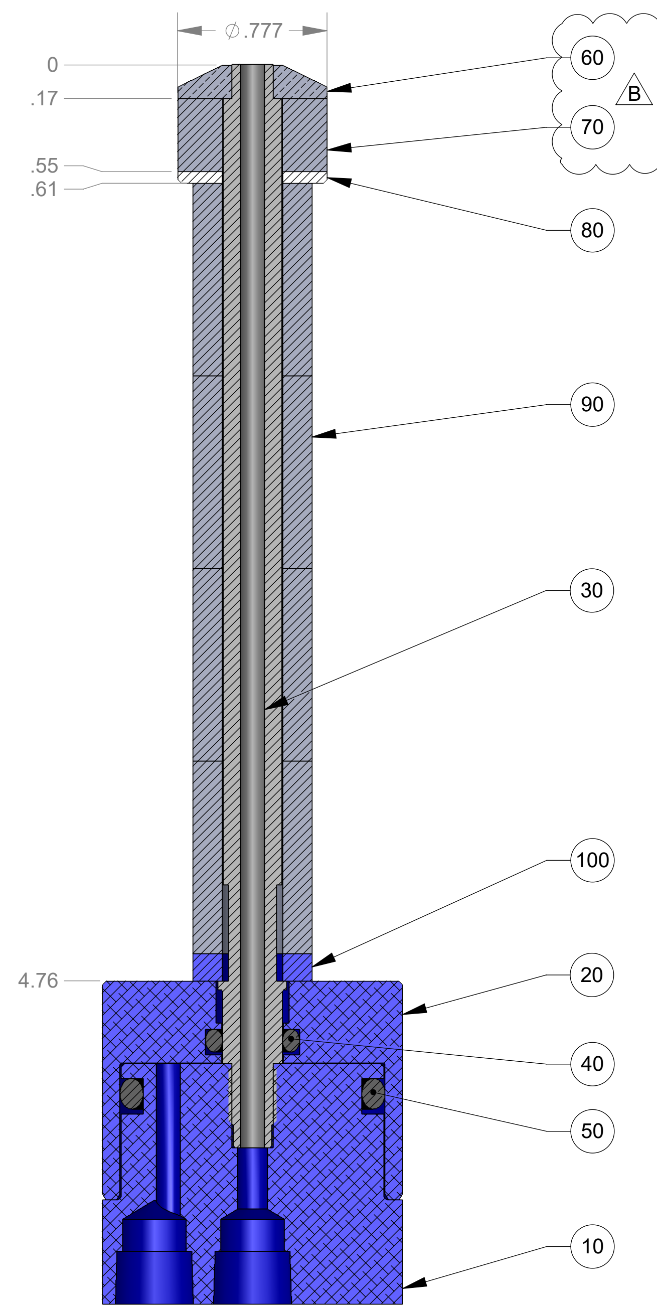
SECTION A-A
