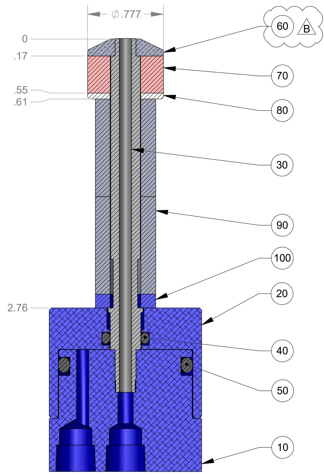
SECTION A-A
