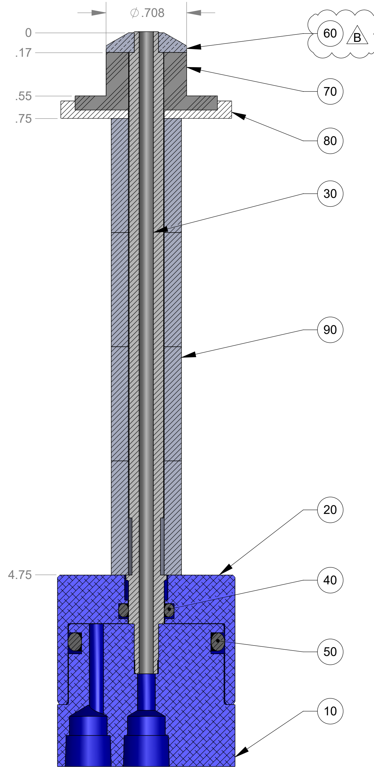
SECTION A-A
