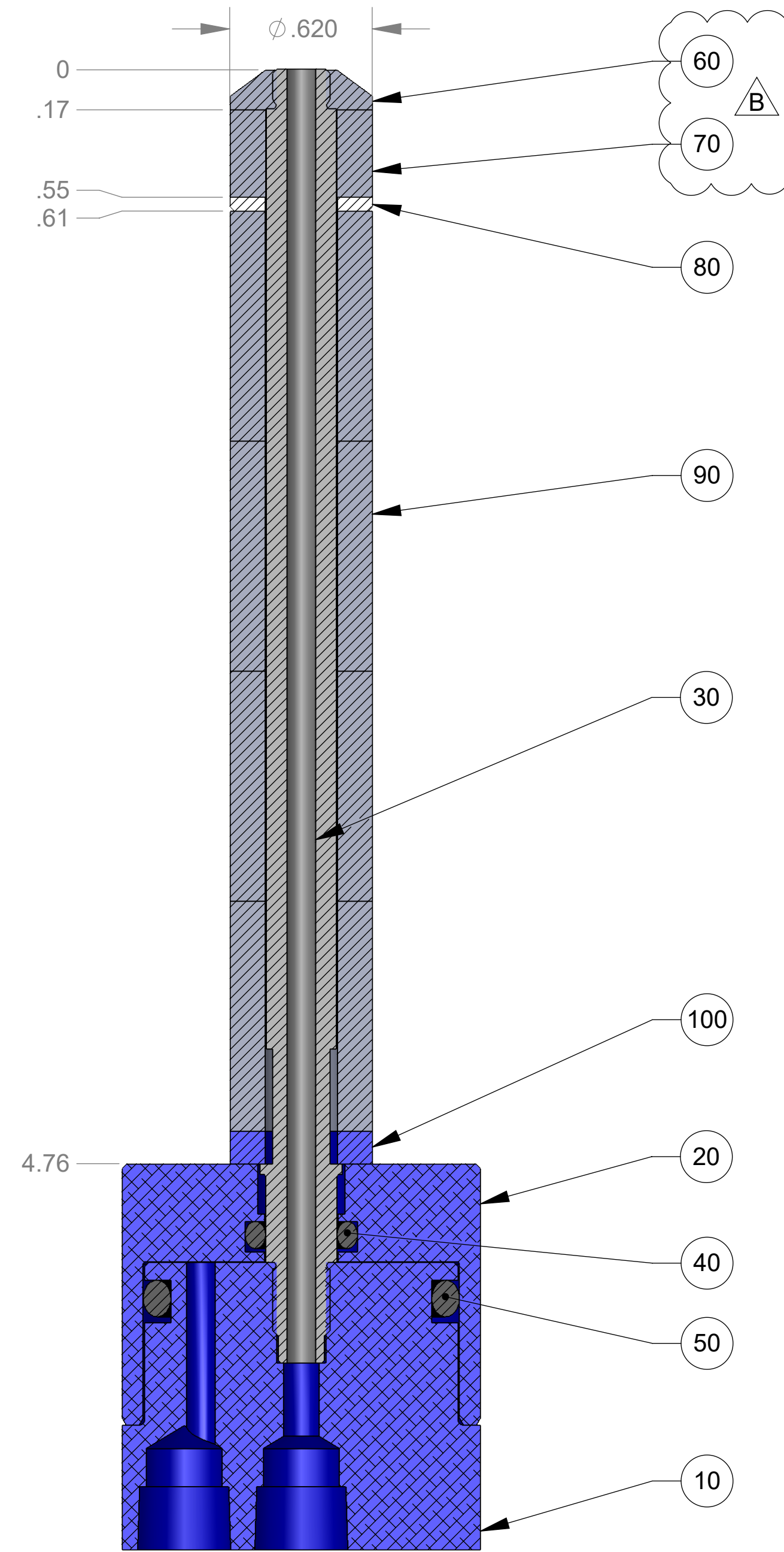
SECTION A-A
