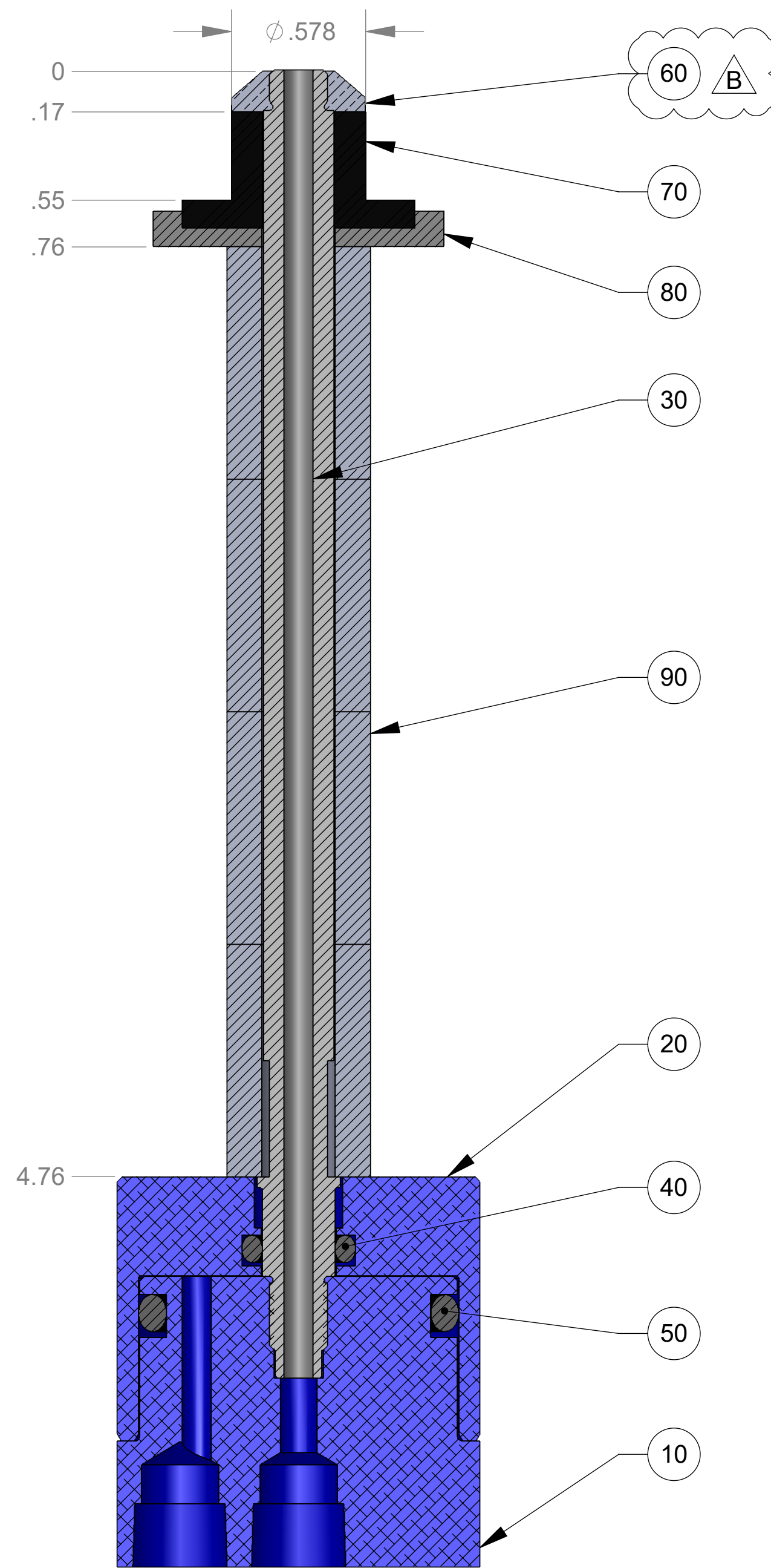
SECTION A-A
