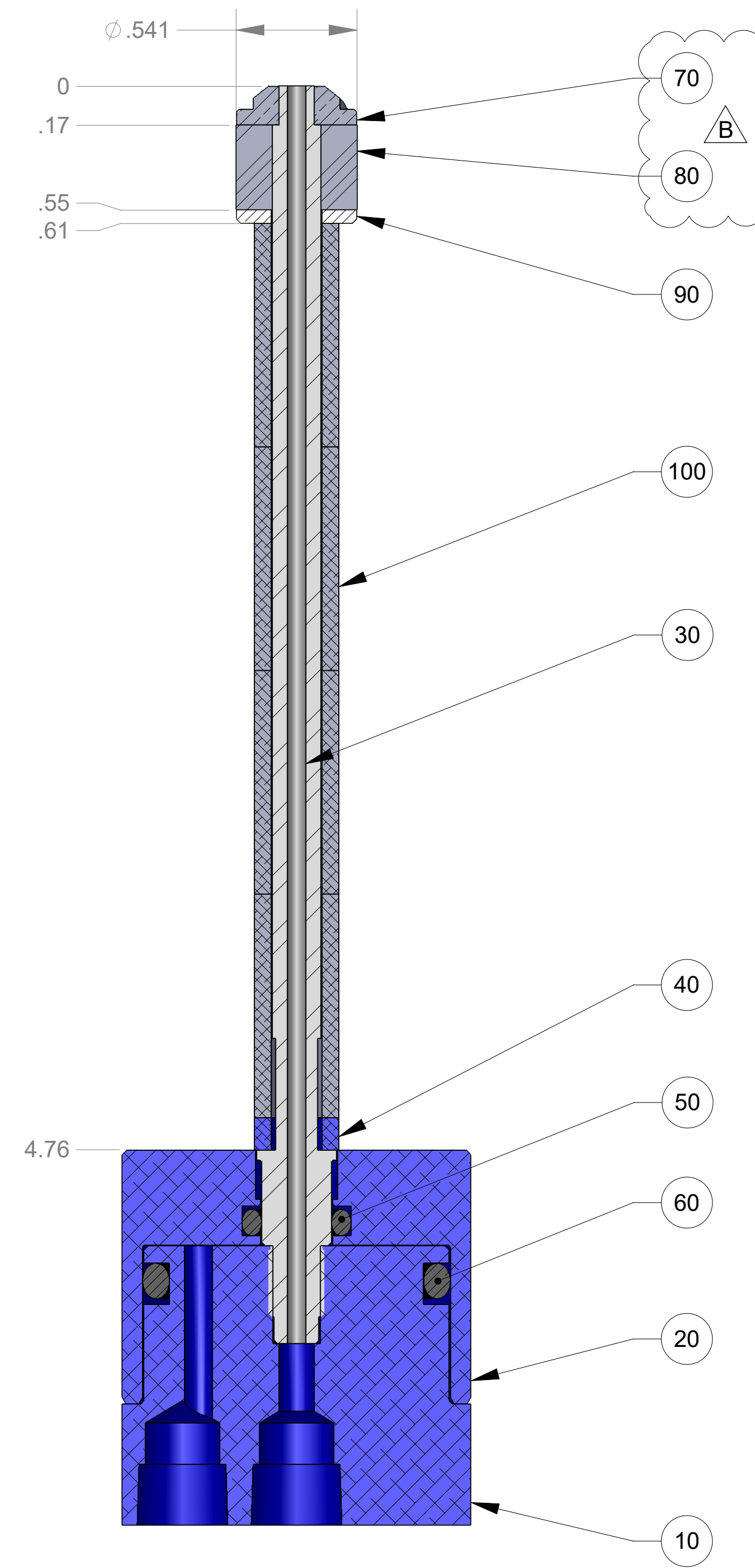
SECTION A-A
