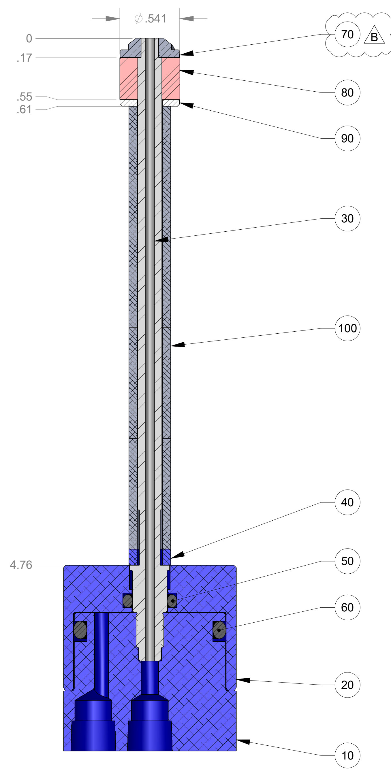
SECTION A-A
