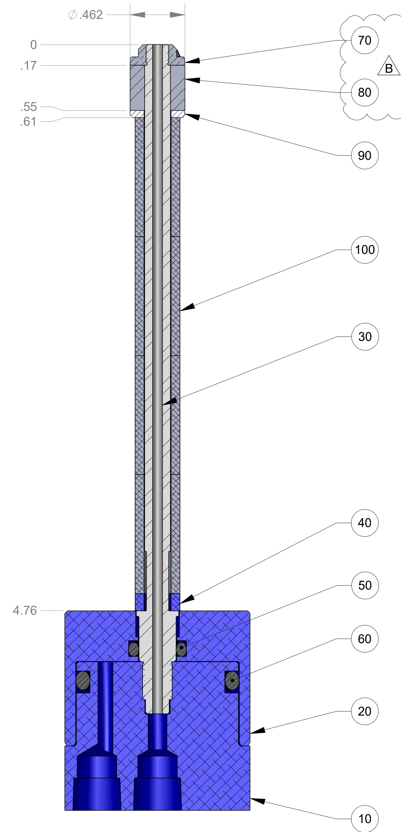
SECTION A-A
