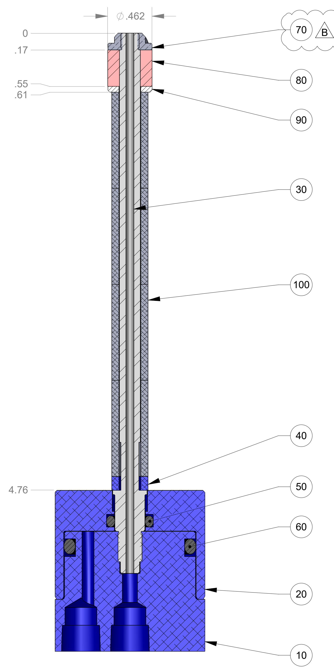
SECTION A-A
