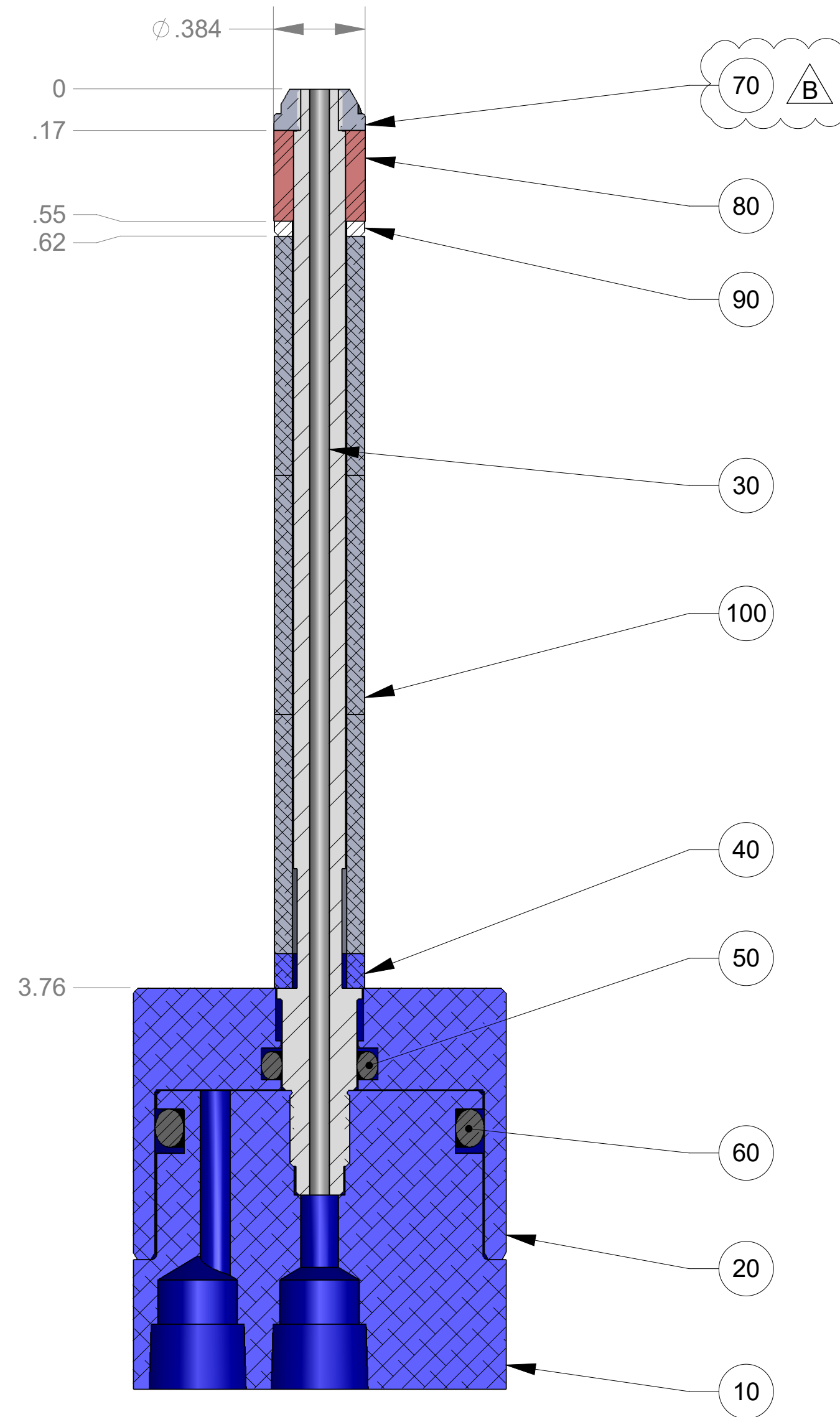
SECTION A-A
