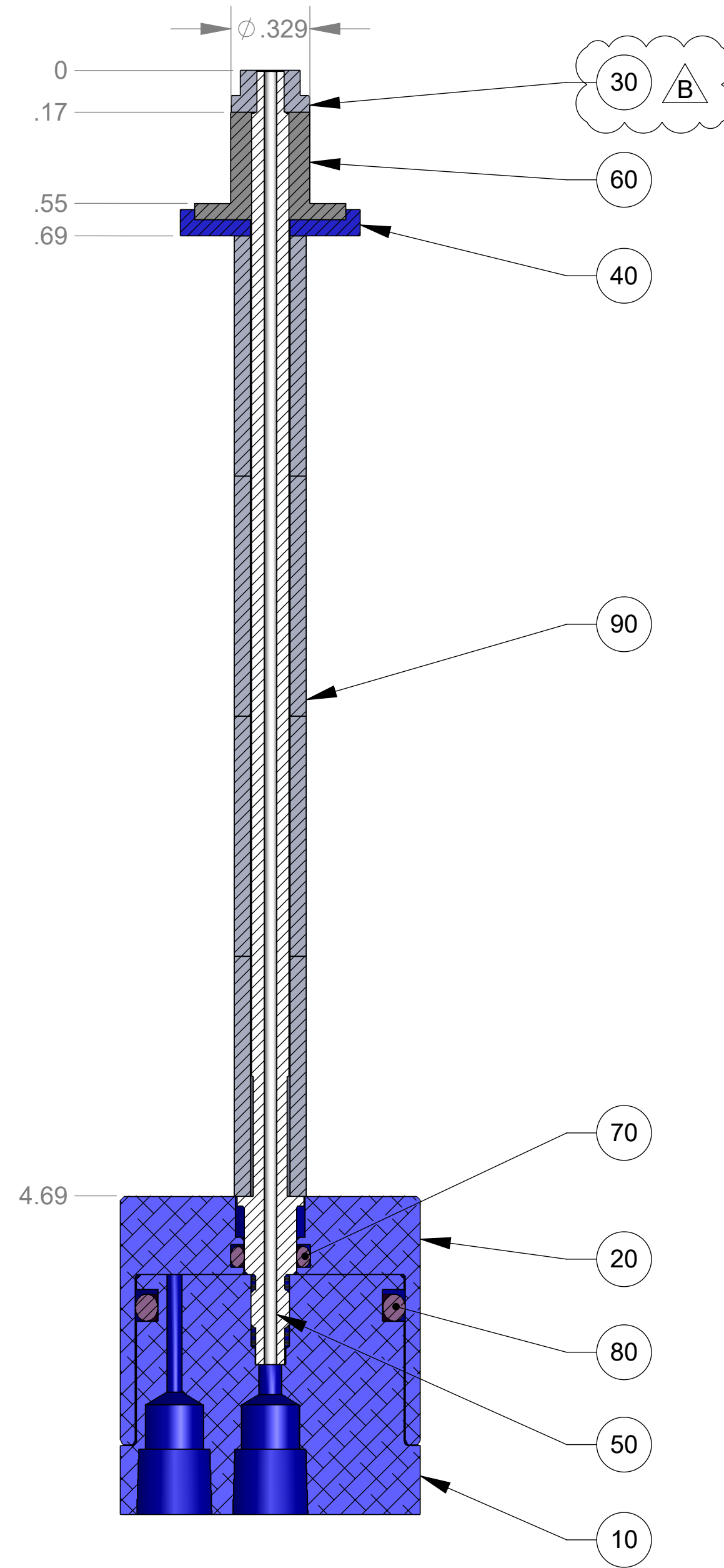
SECTION A-A
