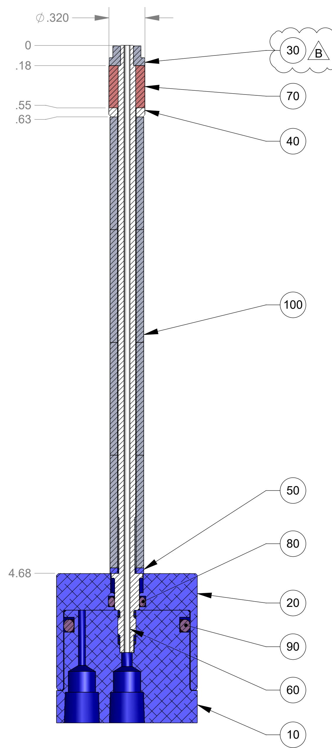
SECTION A-A
