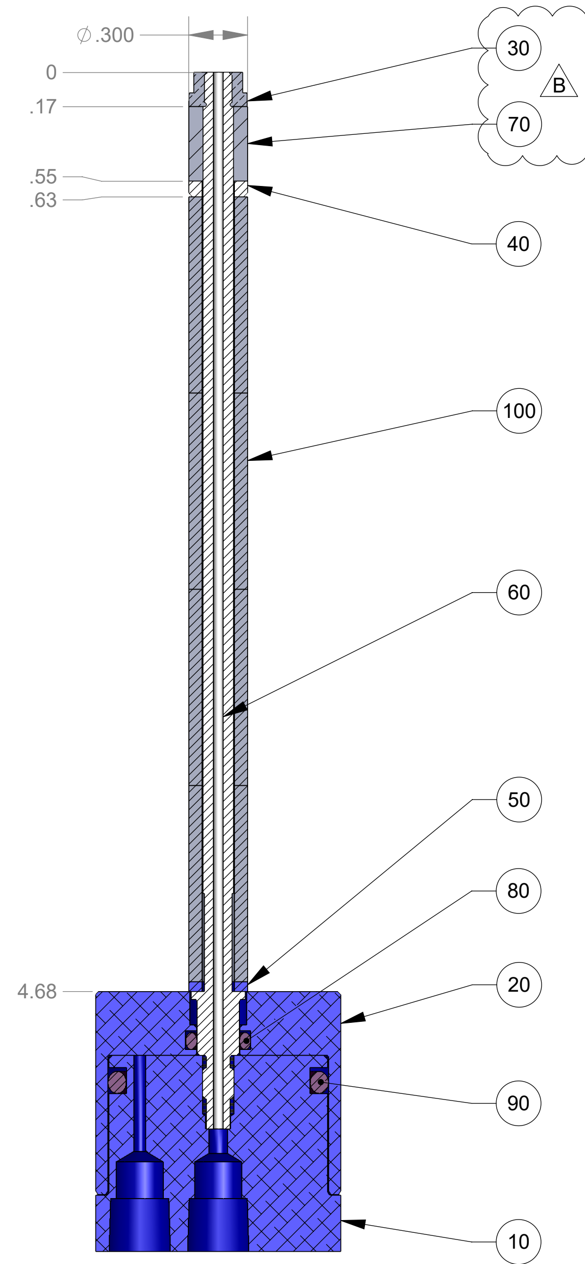
SECTION A-A
