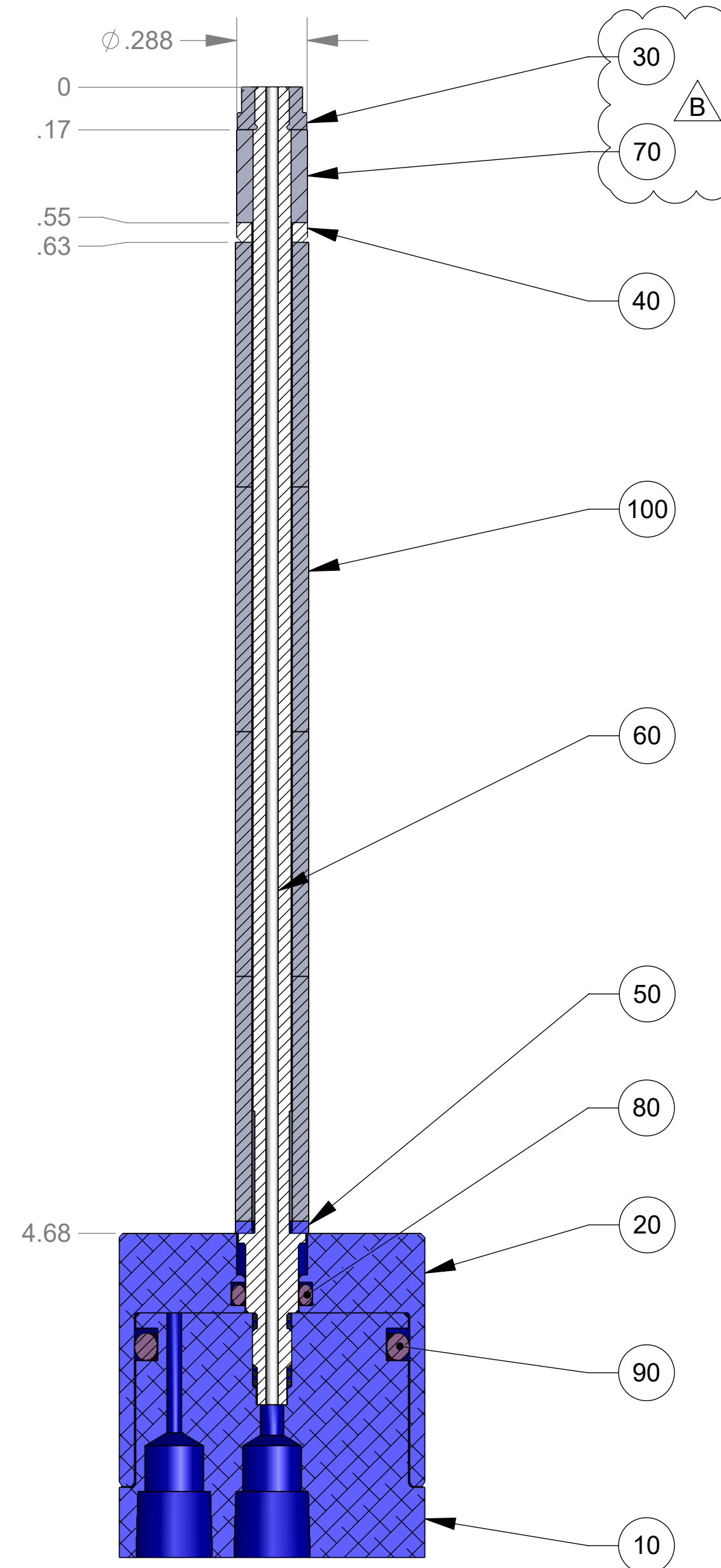
SECTION A-A
