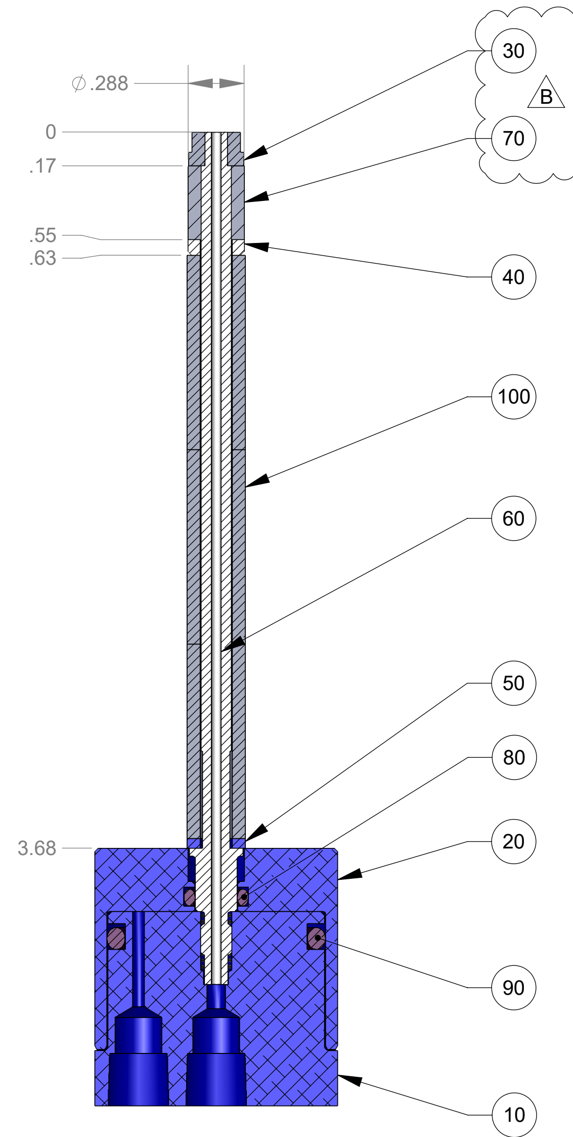
SECTION A-A
