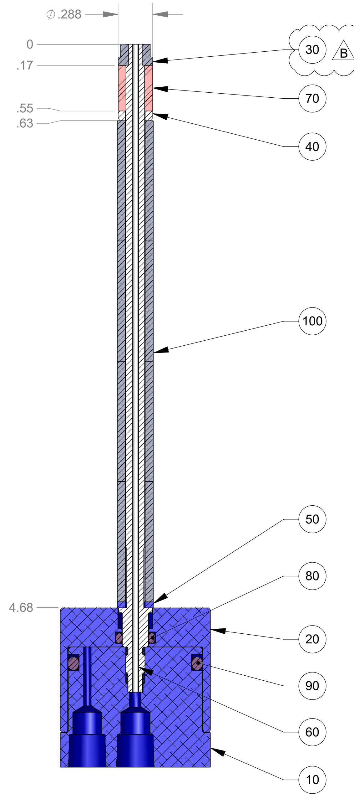
SECTION A-A
