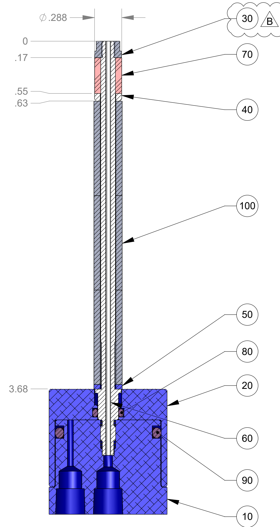
SECTION A-A
