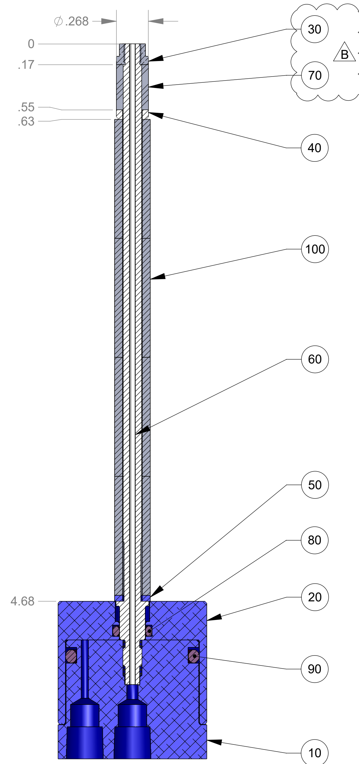
SECTION A-A
