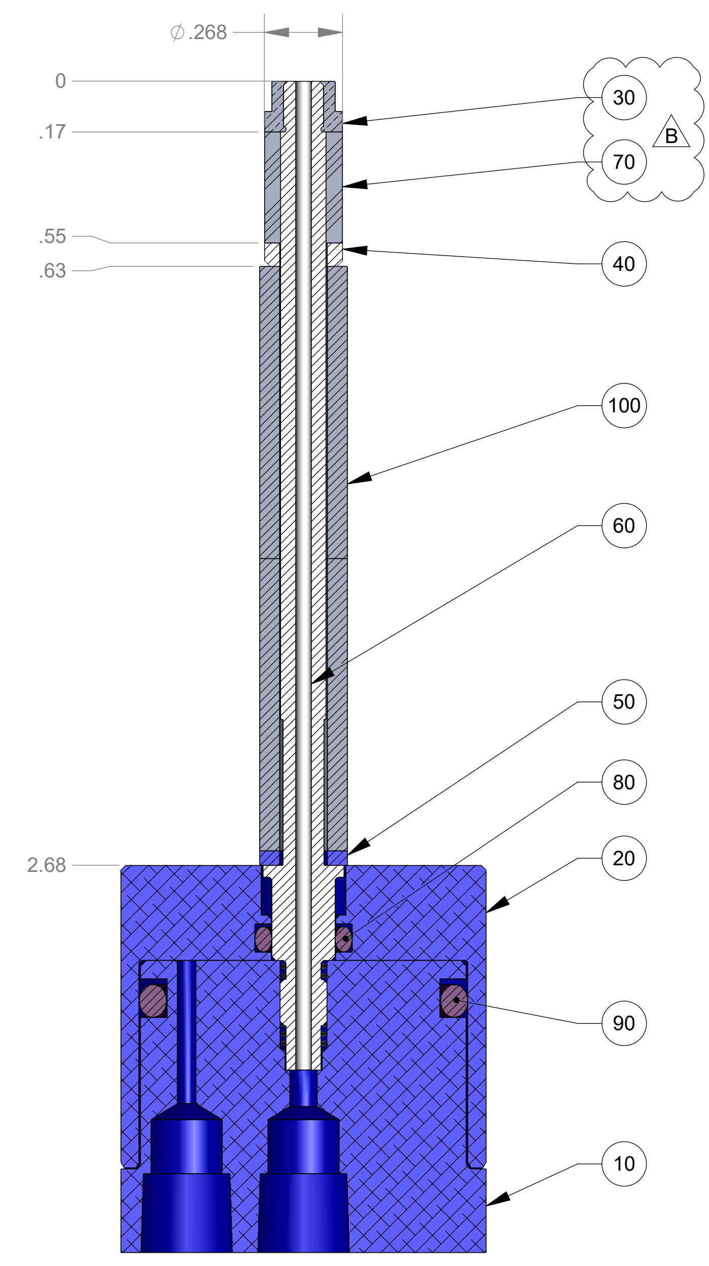
SECTION A-A SCALE 3 : 1
