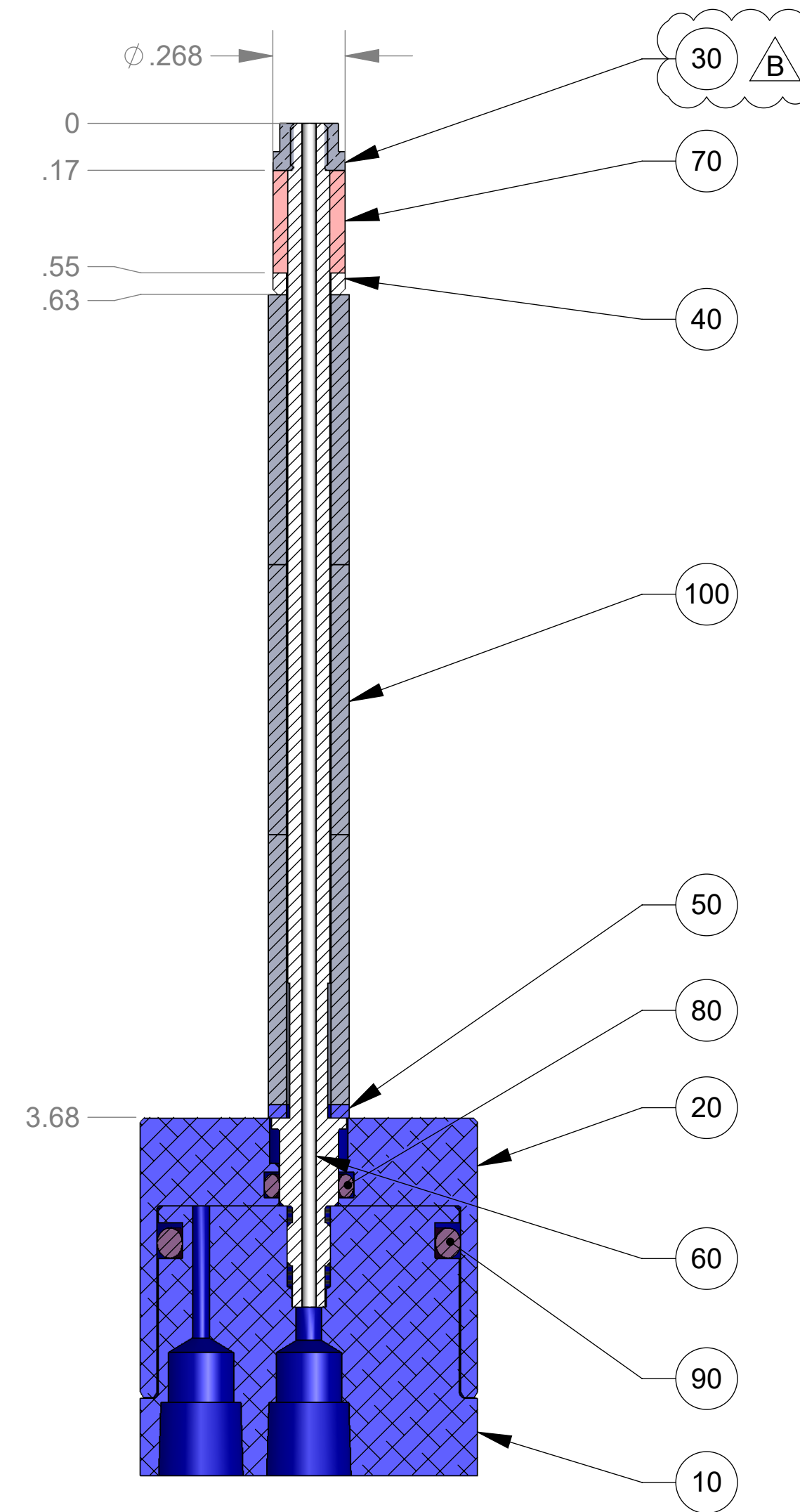
SECTION A-A
